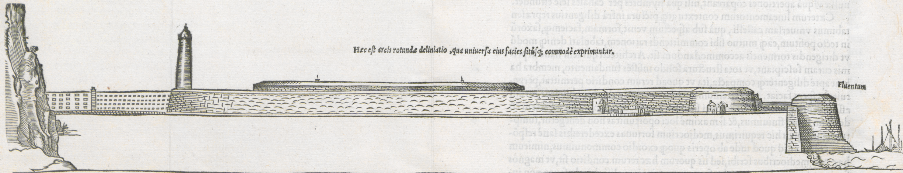
Hic medium arcis eductæ lineamentum exprimitur, itemque fossarum laxitas & altitudo, deinde coclearum, scalarum, portarum, pontium consimiliumque ratio designatur.
