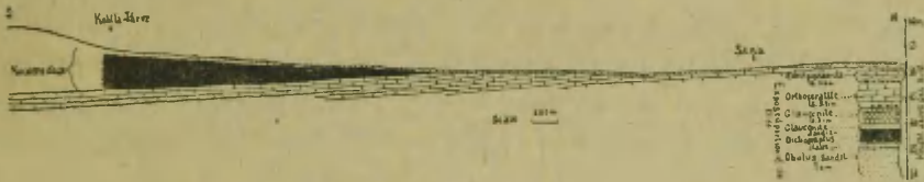
Text fig. 1. Section: Kohtla-Järve — Saka.
