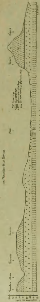
Text fig. 11. Section: Vanamõisa-Püssi-Kukruse.
