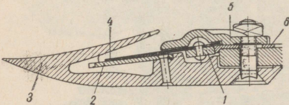
Abb. 2. Schneidwerk eines Grasmähers.
