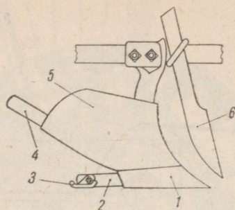
Abb. 5. Teile des Pflugkörpers.
