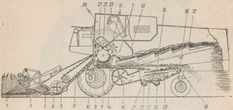
Abb. 1. Der Mähdrescher E 512.
