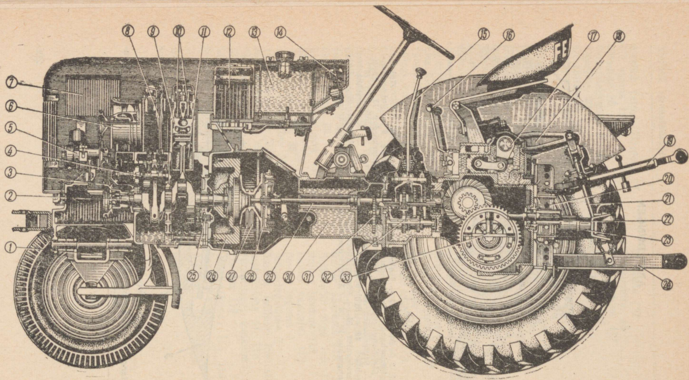
Abb. 3. Der luftgekühlte Traktor F17.
