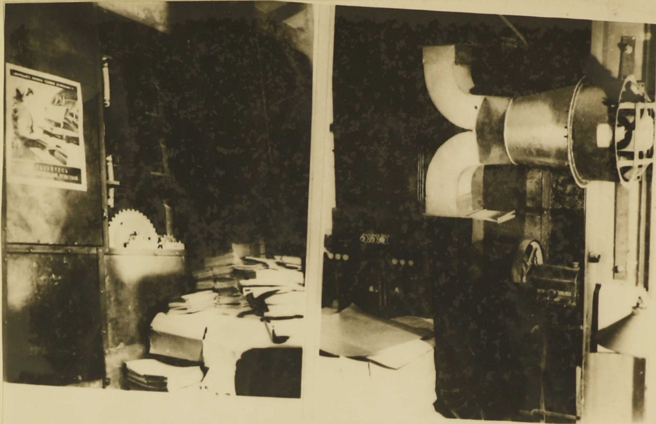
Raamatukaante- ja selja kuivatusseadeldis Kuivatusseadeldise läbilaskevõime on 1100 raamatukaant ja samaaegselt 1400 raamatuplokki (plokk 15pg.) tunnis. Kokkuhoid aastas üle 60 tuh. rubla.
