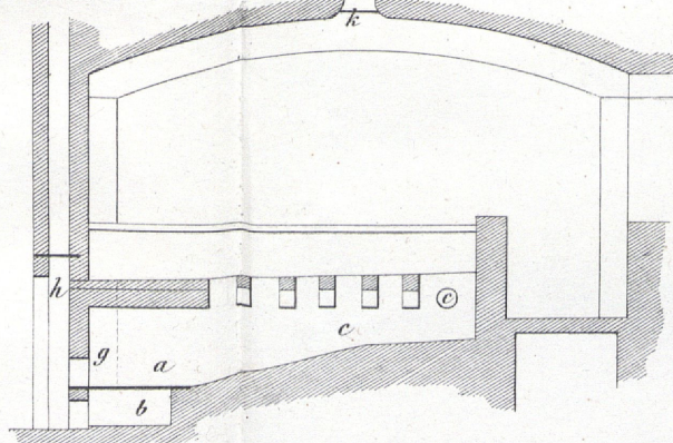
Fig. 130. C. Längendurchschnitt.
