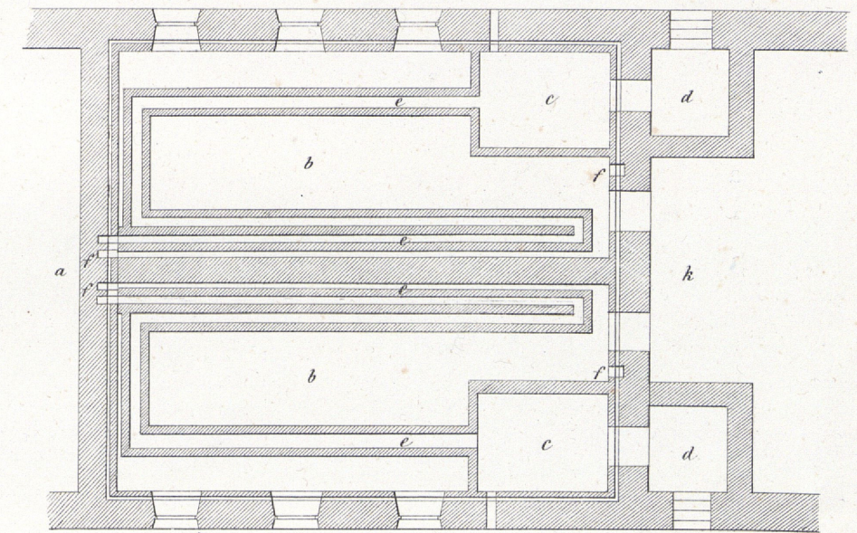
Fig. 125. C. Grundriß.
