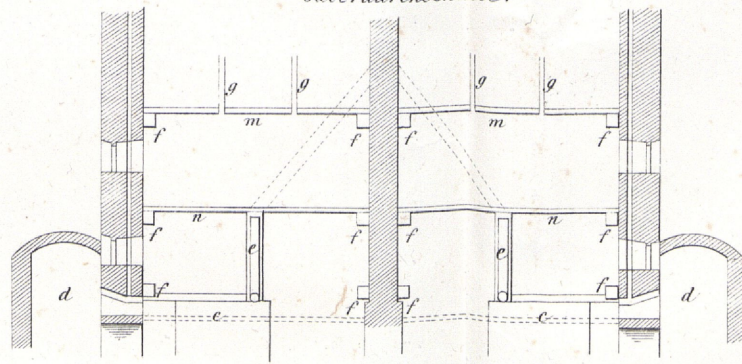
Fig. 124. B. Querdurchschnitt.
