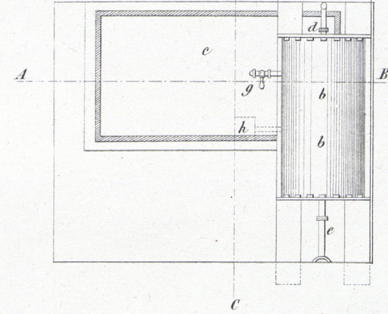
Fig. 132. Grundriss. D.
