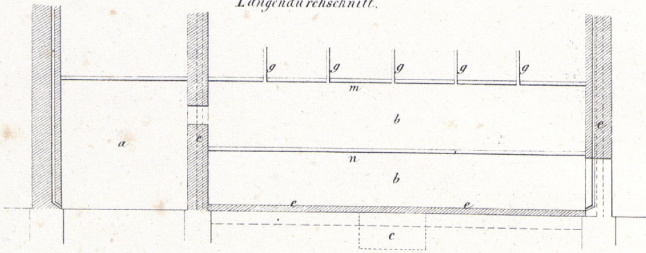
Fig. 124. A. Längendurchschnitt.
