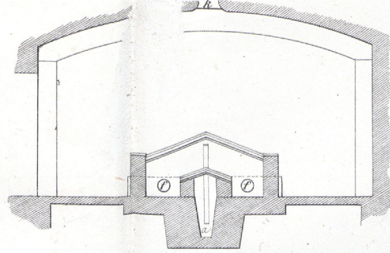
Fig. 130. A. Grundriss.
