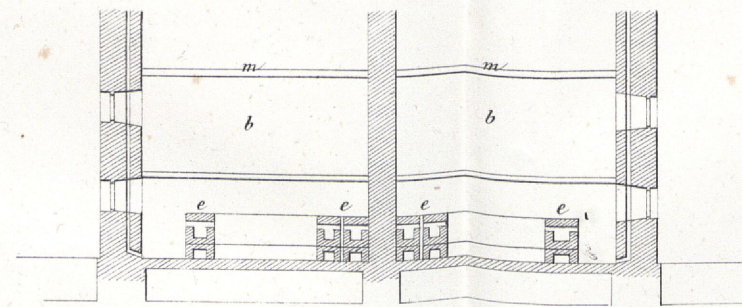
Fig. 125. B. Querdurchschnitt.
