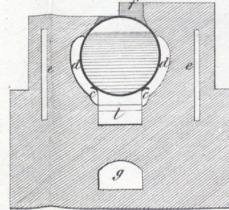
Fig. 131. C. Querdurchschnitt.
