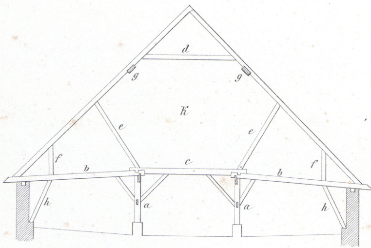
Durchschnitt c.d. ad Fig. 123.
