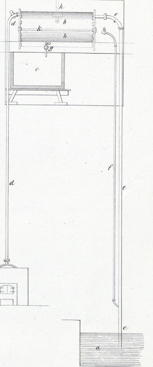
Fig. 132. Durchschnitt nach C D.
