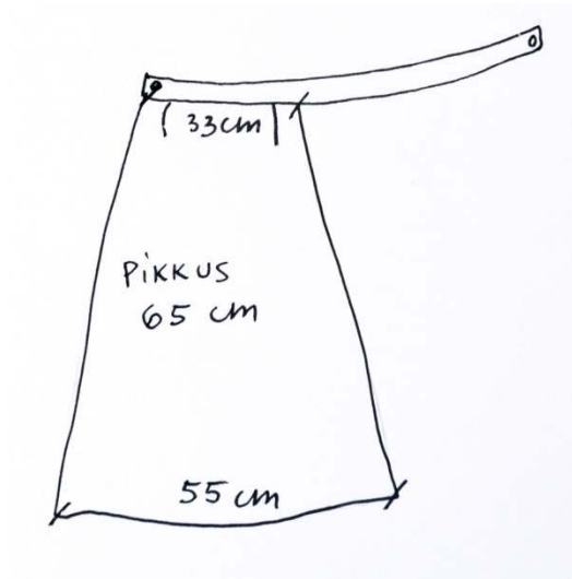
Klassikalise, alt laieneva nööpkinnisega põlle tööjoonis
