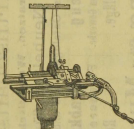
Strickmaschinen.
