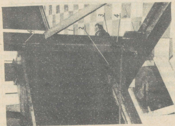
Фиг. 3. 1-стенд испытания, 2-жесткая приладка, 3-винтовая установка для предварительного напряжения, 4-болты, фиксирующие положение балки
