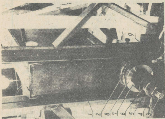
Фиг. 2. 1-торцовое ребро балки, 2-опорная шайба, 3-наконечник затяжки, 4-гайка, 5-шайба, 6-шпилька, 7-натяжная гайка, 8-коробка для подшипника, 9-клюц
