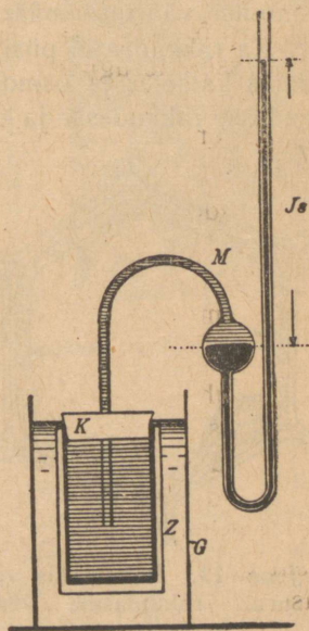
Joon. 12. Osmomeeter.
