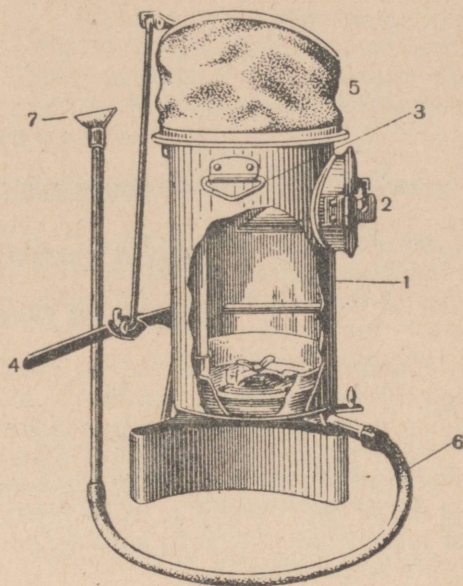
Joon. 24. Tolmuti (osa seinast kõrvaldatud): 1 — tolmuti keha; 2 — ava mürkaine sissepanemiseks; 3 — aas, mille külge kinnitatakse seljakandmise rihmad; 4 — kang, millega pannakse käima lööts (5); 6 — kummitoru; 7 — metalltoru koos mürkaine laialipuistajaga.
