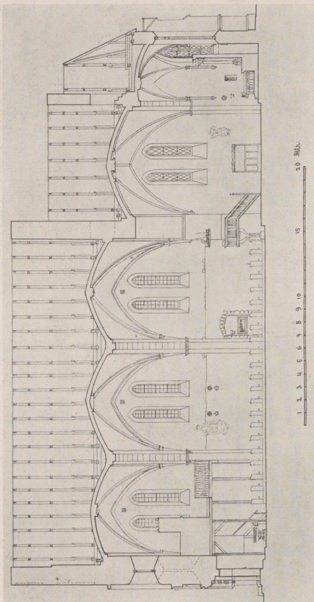
Valjala kirik. Pikkilõige. (N. Paulseni järgi).
