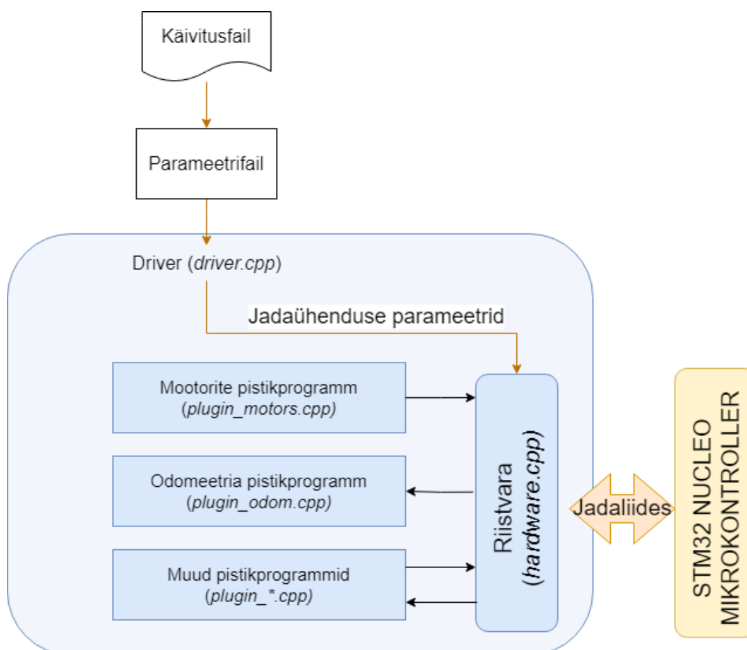
Joonis 2. Robotont ROS1 draiveri arhitektuur
