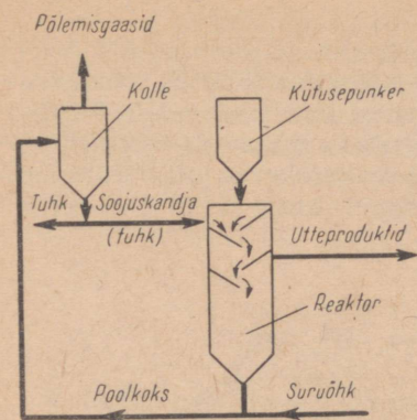
Joonis 50. Põlvkivi termineline töötlemine tahke soojuskandjaga.
