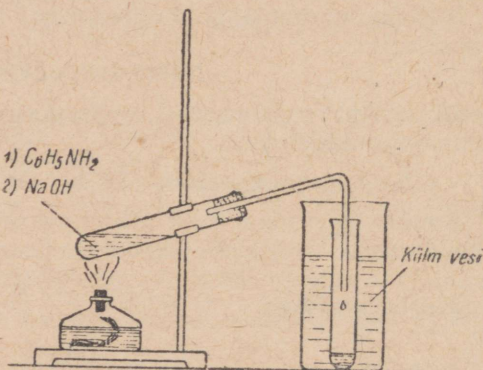
Joonis 80. Nitrobenseeni destilleerimine.
