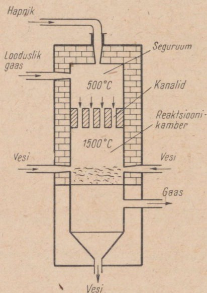
Joonis 23. Reaktor atsetüleeni tootmiseks metaani termooksüdatsioonil.
