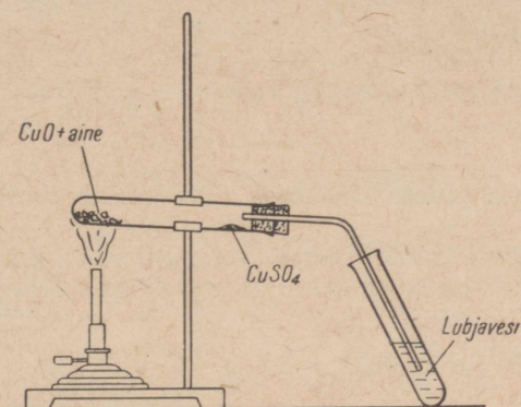
Joonis 85. Orgaanilise aine analüüsideade.
