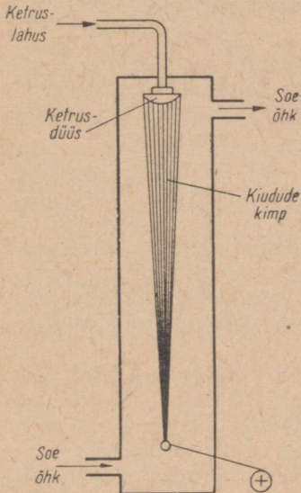
Joonis 78. Atsetaatsiidi tootmine.
