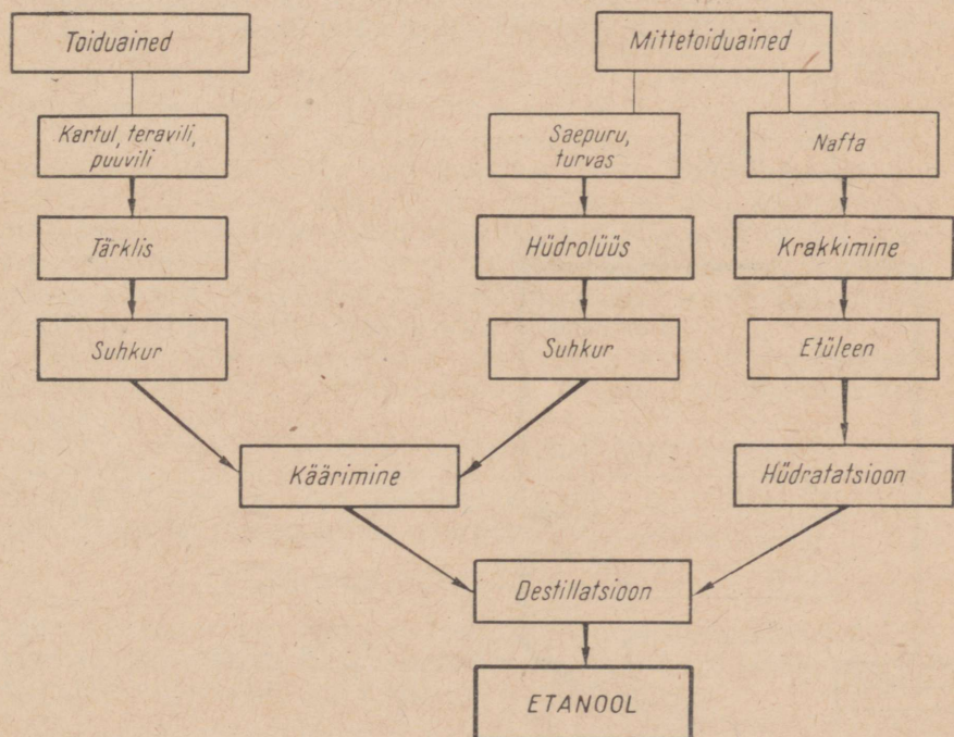
Joonis 55. Etanooli saamine.
