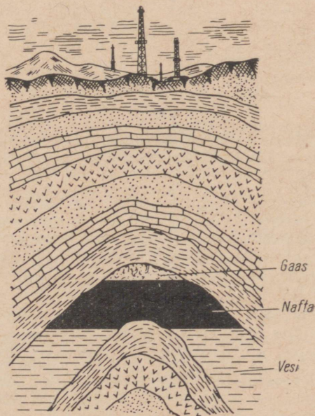
Joonis 31. Nafta leiukoha geoloogiline läbilõige.
