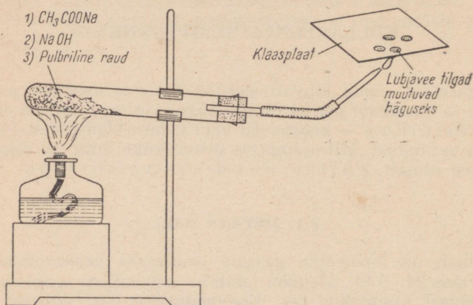
Joonis 2. Metaani põlemisel tekib veeaur ja süsinikdioksiid.
