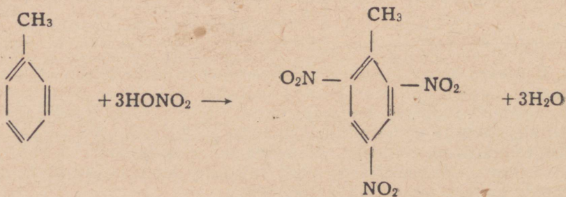
trinitrotolueen
