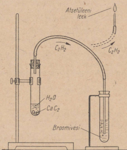
Joonis 21. Atsetüleeni saamine ja omadustega tutvumine.
