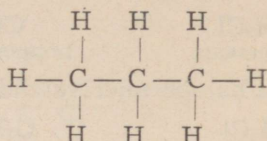
propaani struktuurivalem
