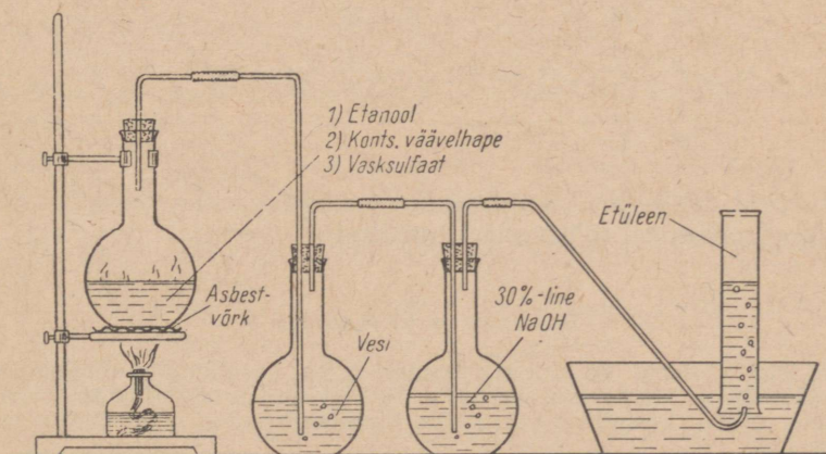
Joonis 8. Etüleen saamine etanoolist.
