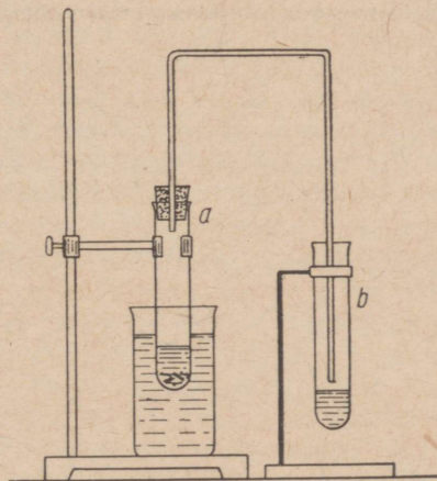
Joonis 25. Bromobenseeni saamine.
