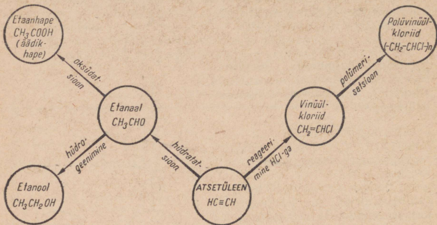
Joonis 83. Atsetüleenist saadavate produktide edasise töötlemise võimalusi.
