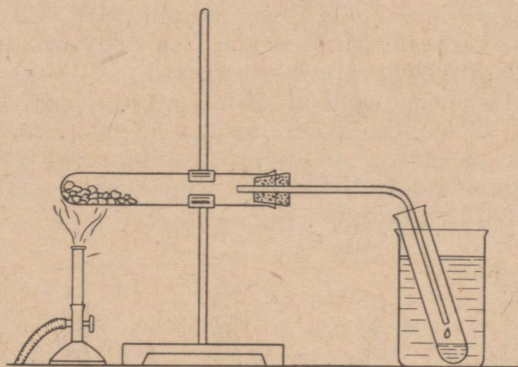
Joonis 27. Stürooli depolümeriseerimine.
