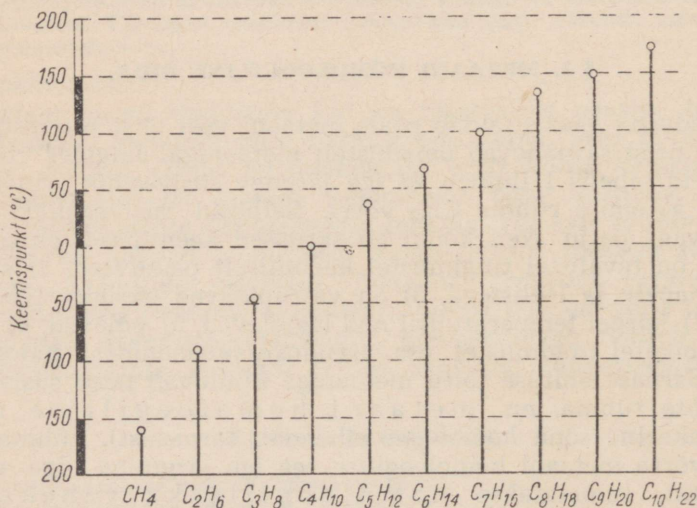
Joonis 4. Küllastunud süsivesinike keemispunkti sõltuvus nende koostisest.
