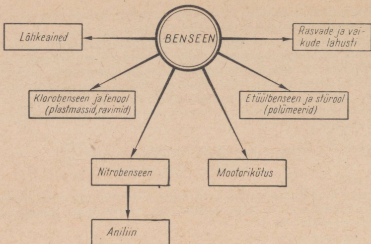
Joonis 26. Benseeni kasutamine.
