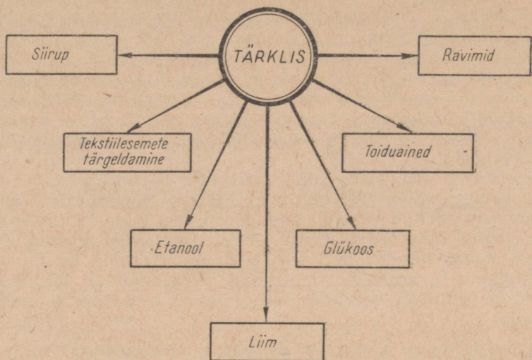
Joonis 72. Tärklise kasutusalasid.
