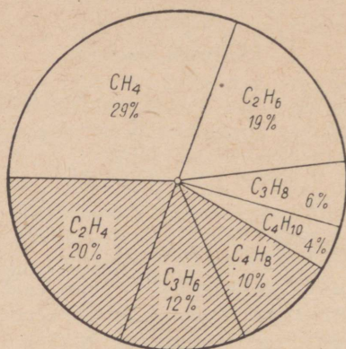
Joonis 9. Nafta krakkgaaside keskmine koostis.
