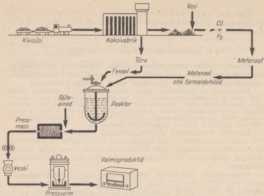
Joonis 62. Fenoolformaldehüüdvaikude tootmine.
