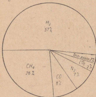
Joonis 45. Koksigaasi keskmine koostis.
