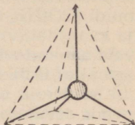
Joonis 6. Süsiniku aatomi tetraaeder.
