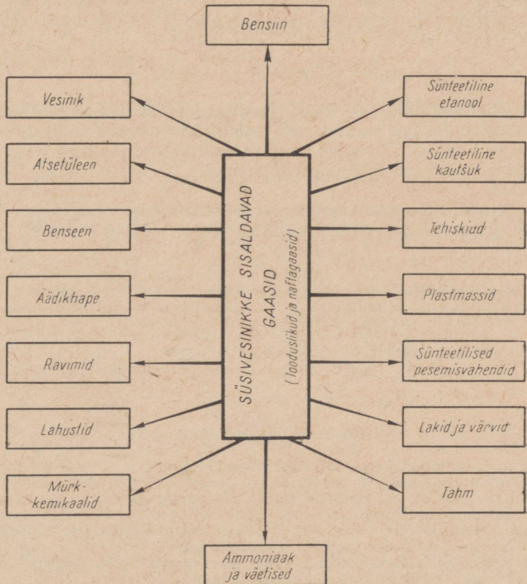
Joonis 33. Looduslike gaaside kasutusalasid.
