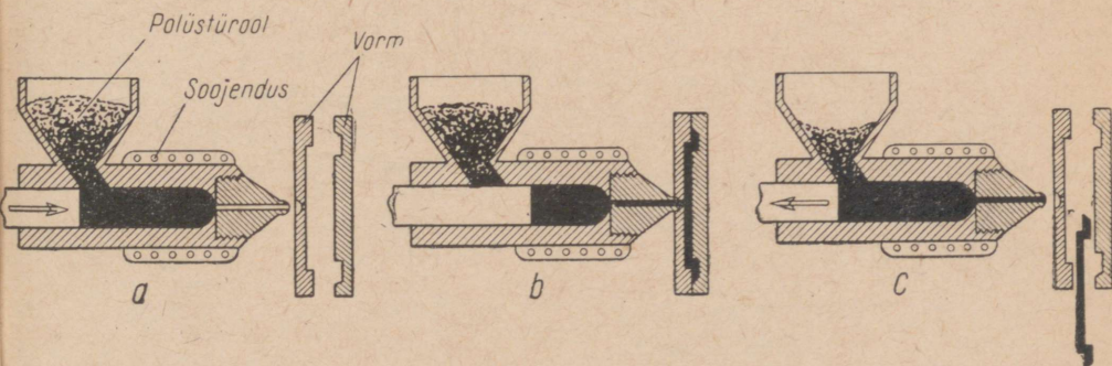
Joonis 29. Press rõhu all valamiseks.
