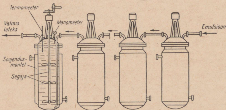
Joonis 28. Polümerisaatorite patareid.
