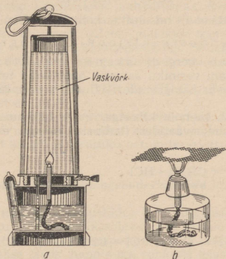
Joonis 3. Kaevurilamp (Davy lamp): a — lamp lõikes; b — leek ei läbi võrku.
