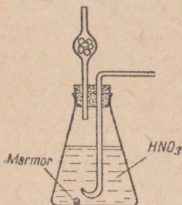
Joonis 84. Kaltsiumkarbonaadi sisalduse määramine marmoris.
