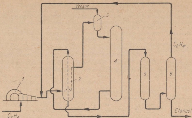
Joonis 57. Etanooli tootmine etüleenist:
