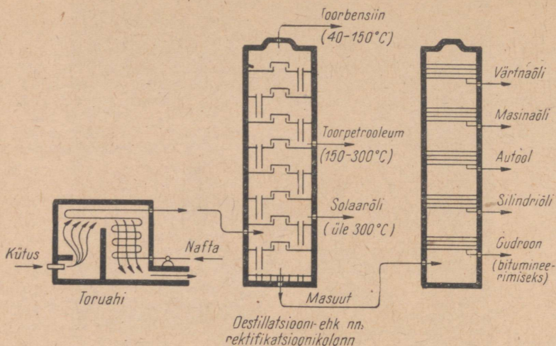
Joonis 40. Nafta rektifikatsioonikolonn skeem.
