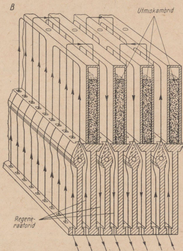
Joonis 44. Koksiahi.
