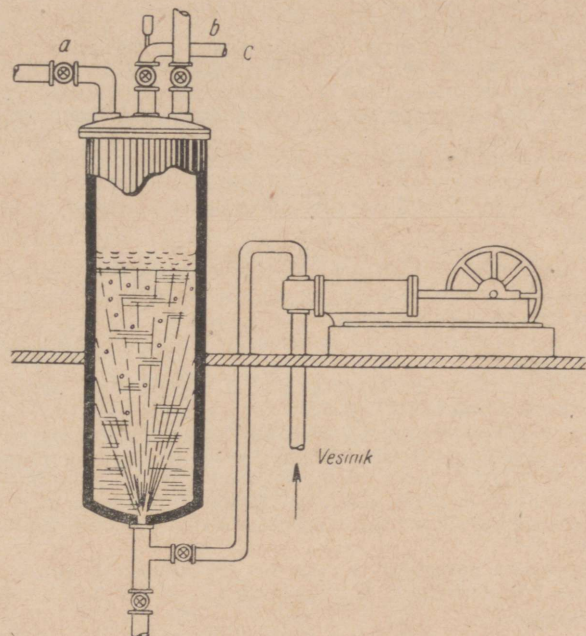
Joonis 65. Rasvade hüdrogeenimise seade:
