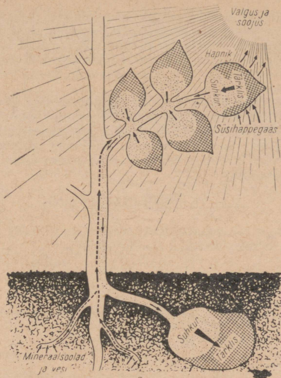
Joonis 68. Süsivesikute süntees ja ladestumine taimedes.
