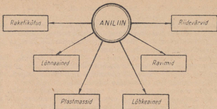
Joonis 81. Aniliini kasutusalasid.
