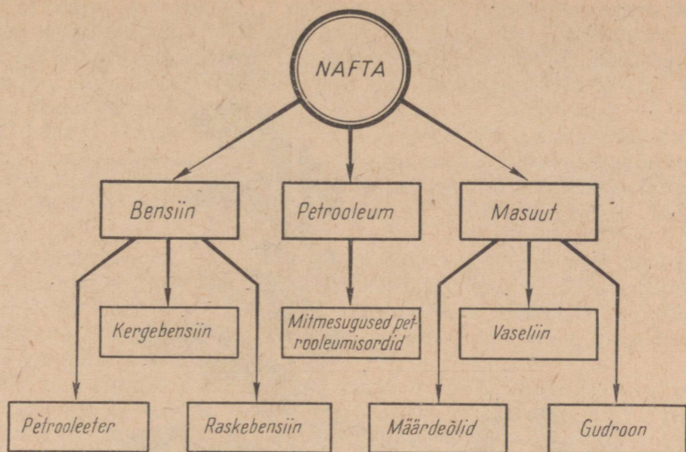
Joonis 42. Nafta fraktsioneerimise saadused.
