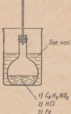
Joonis 79. Nitrobenseeni taandamine.
