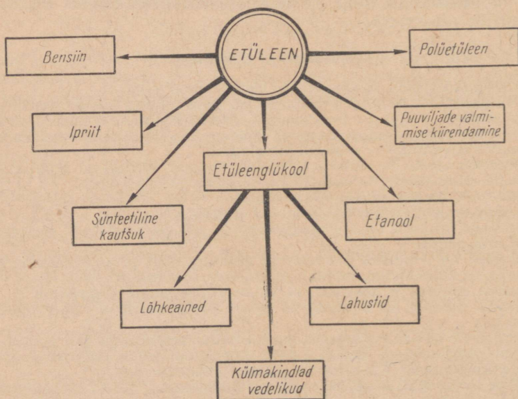
Joonis 7. Etüleen kasutamine.
