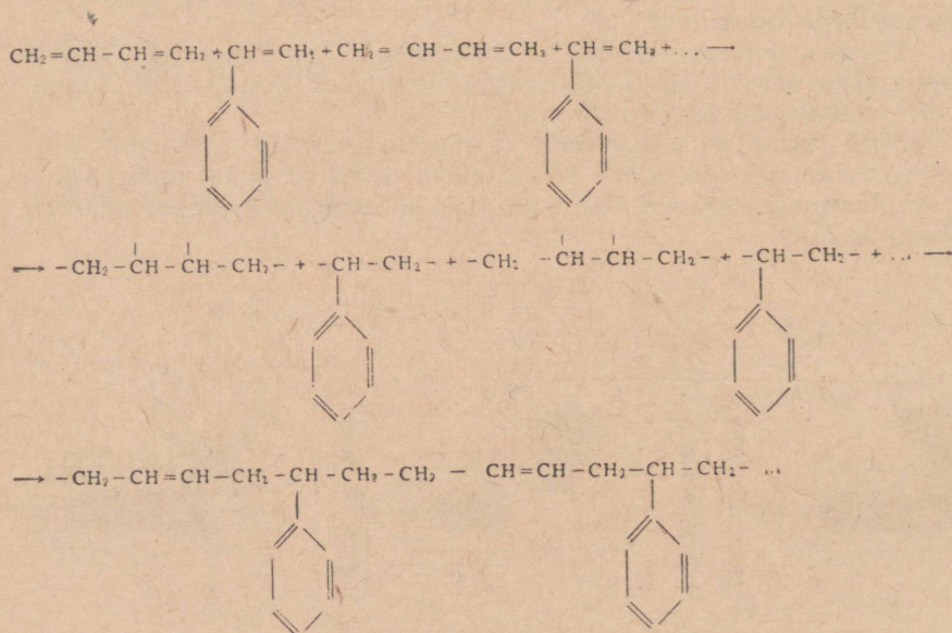
butadieenstürool kautšuk
