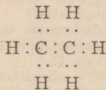
etaan
