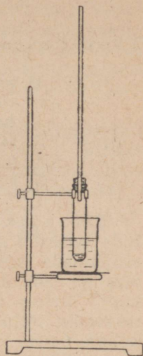
Joonis 87. Rasvade ekstraheerimine.
