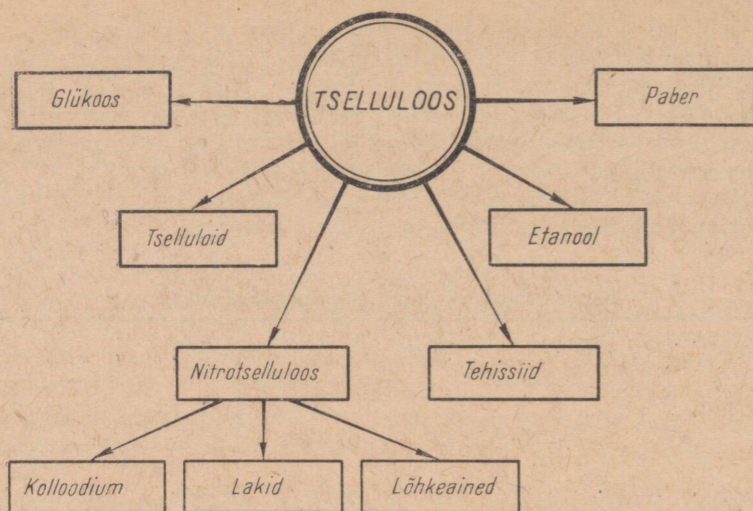
Joonis 73. Tselluloosi kasutusalasid.
