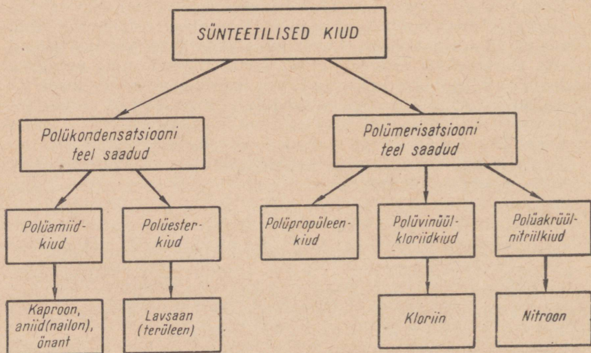
Joonis 74. Kiudainete klassifikatsioon.
