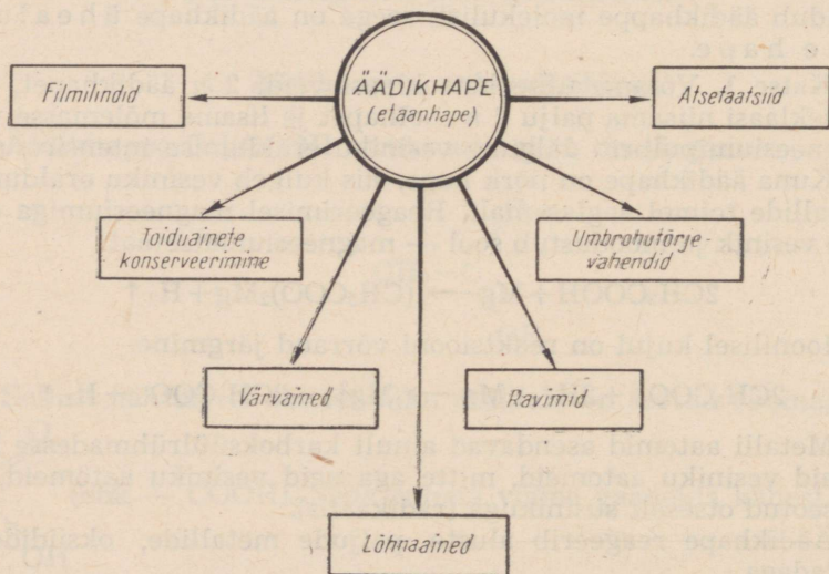
Joonis 63. Äädikhappe kasutusalasid.
