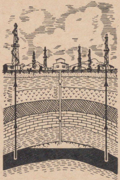
Joonis 35. Nafta tungimine maapinnale gaaside või suruõhu kasutamise tõttu.
