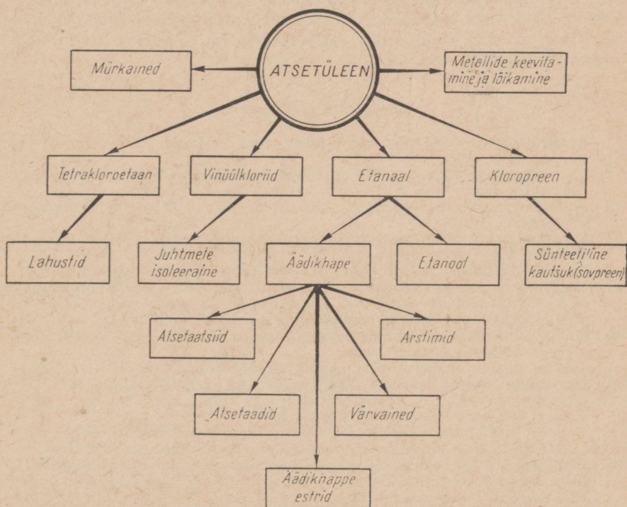
Joonis 24. Atsetüleenil kasutamine.
