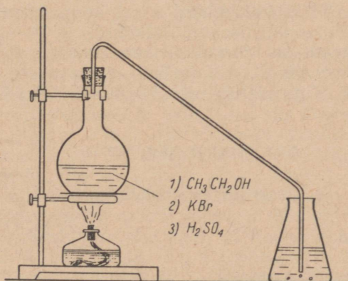
Joonis 86. Bromoetaani saamine.
