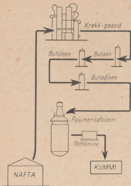
Joonis 17. Sünteetilise kautšuki tootmine naftaproduktidest B. Bözovi meetodil.
