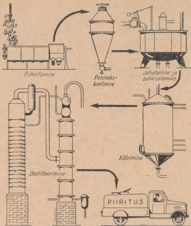
Joonis 71. Etanooli (piirituse) tootmine kartulitest.
