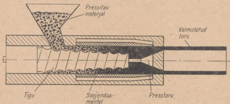
Joonis 10. Polüetüleeneseemete valmistamine rõhu all valamisel.
