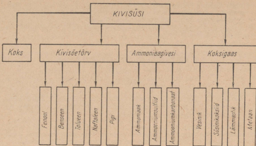
Joonis 46. Kivisöe koksistamise saadused.
