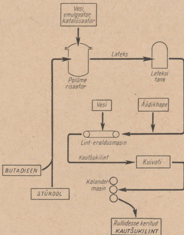
Joonis 30. Butadieenstüroolkautšuki tootmise skeem.
