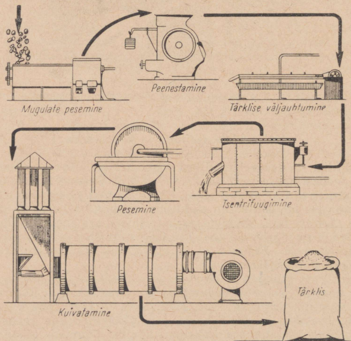
Joonis 69. Tärglise valmistamine kartulitest.
