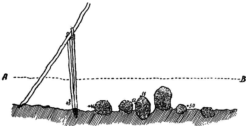
Abb. 12. Profil AB der Herdstelle. ---- Bodenoberfläche. Die von einer gebrochenen Linie umrissenen Steine liegen ausserhalb des eigentlichen Profils. ● — Funde entsprechend denen auf dem Plan Taf. II. Schraffiert sind die tatsächlich gefundenen Reste von Pfählen, das übrige rekonstruiert.
