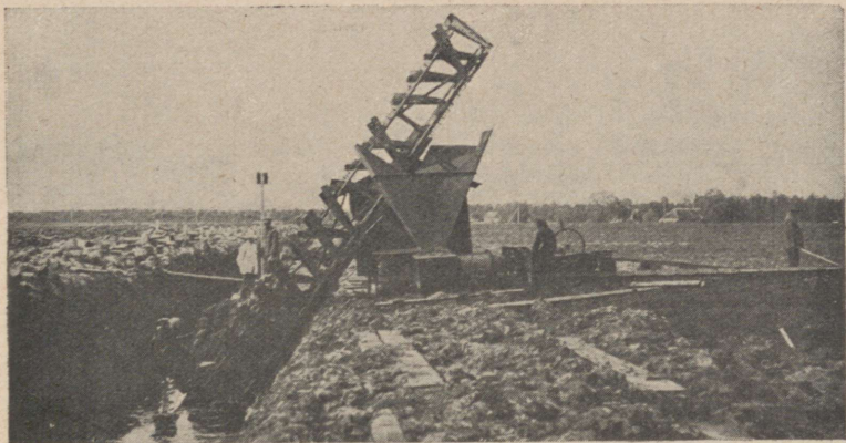
70. joon. Lavassaare (Jõõpre) turbatööstus Pärnumaal. Turba baggermasin töötamas.
