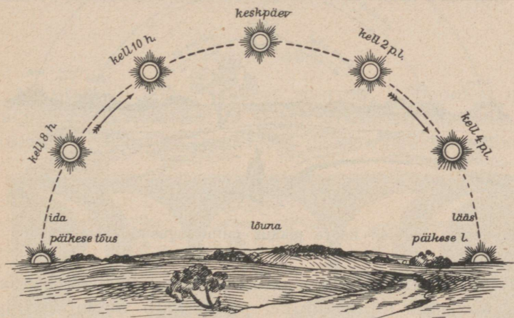
5. joon. Päikese seis päeva jooksul.
