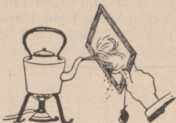
36. joon. Aur muutub veeks.
