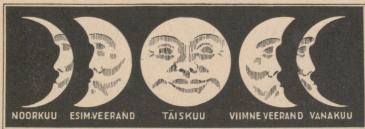
8. joon. Kuu nähted.
