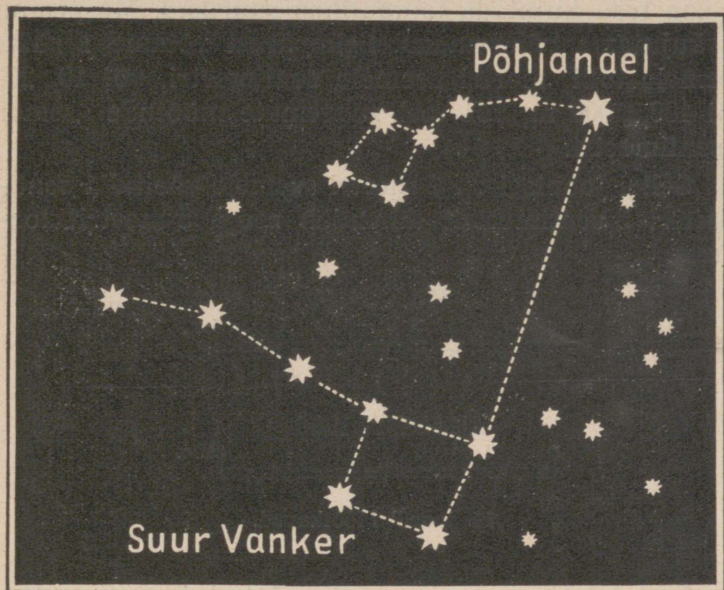
9. joon. Suur Vanker ja Põhjanael.
