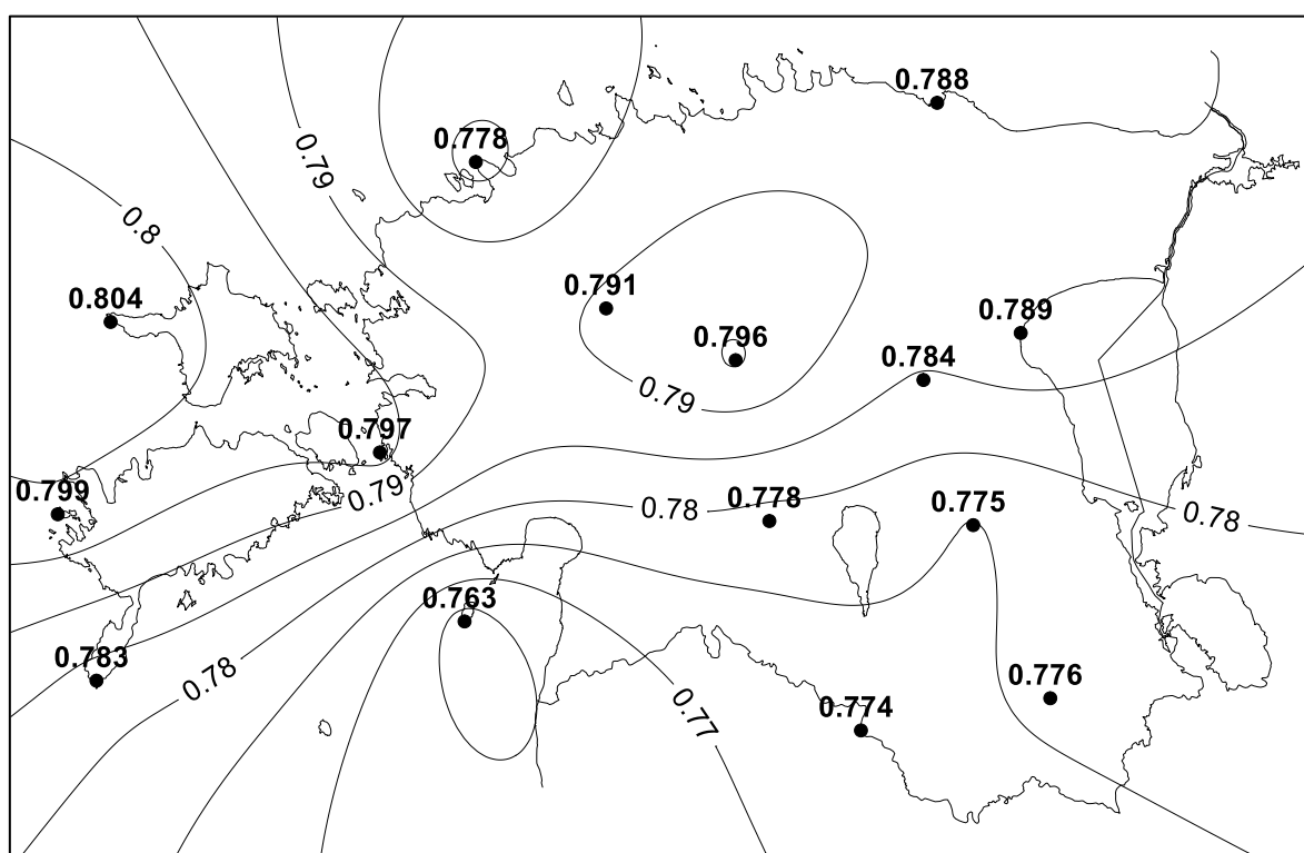
Joonis 11. Talve keskmise maksimaalse temperatuuri ja talvise NAOPC vaheliste korrelatsioonide territoriaalne jaotus perioodil 1951–2015.
