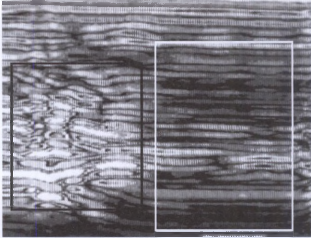
Joonis 2. Joonis 2. Läbilõige kirikumüürist. Selgesti on eraldatavad erineva intensiivsusega peegeldusalad. Valge + hall vasakus servas (mustas ruudus) viitab karbonaatkivimitest müüriosale; hall + must viirutus (valges ruudus) aga osutab kas tühimikule müüris või näiteks krohvialusele puitkonstruktsioonile. Sagedus 500 MHz.
