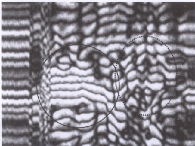
Joonis 1. Hauaplatsi ristiprofiil. Vasakul on näha säilinud kiristu selge peegeldus (täisjoonega ovaal), paremal vanema matuse küsitav jälj (punktir-ovaal). Sagedus 500 MHz.
