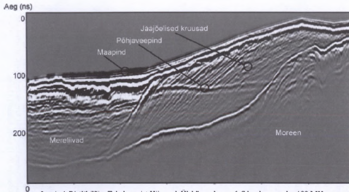
Joonis 4. Ristlâbilõige Tubala oosist Hiiumaal. Ülekõrgendus on 6–7 kordne, sagedus 100 MHz.
