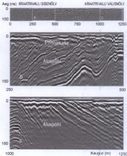
Joonis 3. Läbilõige üle Kärkla kraatri valli, Paluküla. Aluspõhja sisemised peegeldused (a) näitavad, et valli kõrgeim osa on kaugustel 300–850 m. Vahemikus 250–500 m (b) on näha aluspõhja astmelist reljeefi pinnakatte all. Profili lõpus (c) on näha aluspõhja kihtide kallakuse vähenemine vallist kaugenedes. Joonise ülemisel osal on ülekõrgendus 10–12 korda, alumistel 9 korda.
