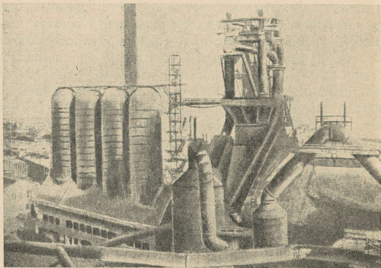
Доменные печи Кузнецкого металлургического завода.
