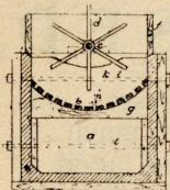
Kartulipesemise masin.
