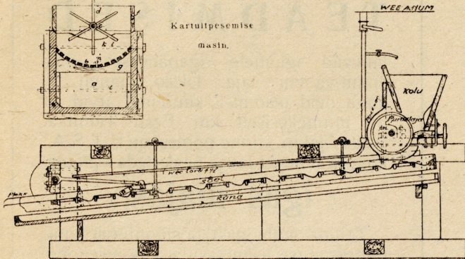
Kartulipurustaja Pikuti läbilõige
