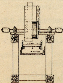
Kartulipurustaja (Põklõige)
