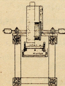
Kartulipurustaja (Põikõige).
