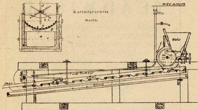
Kartulipurustaja. Pikkvõlliõige
