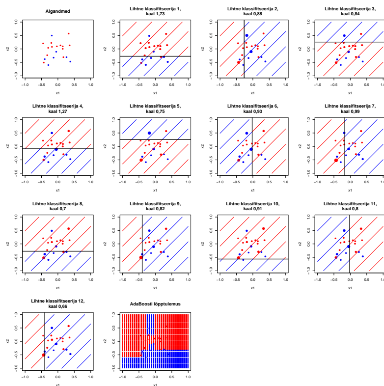
Joonis 4.3: AdaBoost rakendatuna kahemõõtmelisest normaaljaotusest genereeritud juhuslikult klassifitseeritud andmetele. Lihtsa klassifitseerijana on kasutatud otsustuspuud 1 lõikamise ja 2 reeglga (joonistel tähistatud musta sirgega): igal sammul on proovitud kõiki 2 \times 20 = 40 erinevat tulemust andvat klassifitseerijat, mille hulgast on valitud parim. Punktide suurus näitab igal sammul objekti kaalu, viirutatud ala värv näitab, millisesse klassi lihtne klassifitseerija andmed igal iteratsioonil klassifitseeris. Lõpptulemus on lihtsate klassifitseerijate kombinatsioon. Näeme, et AdaBoost eraldab klassid antud andmetel 12 sammuga.
