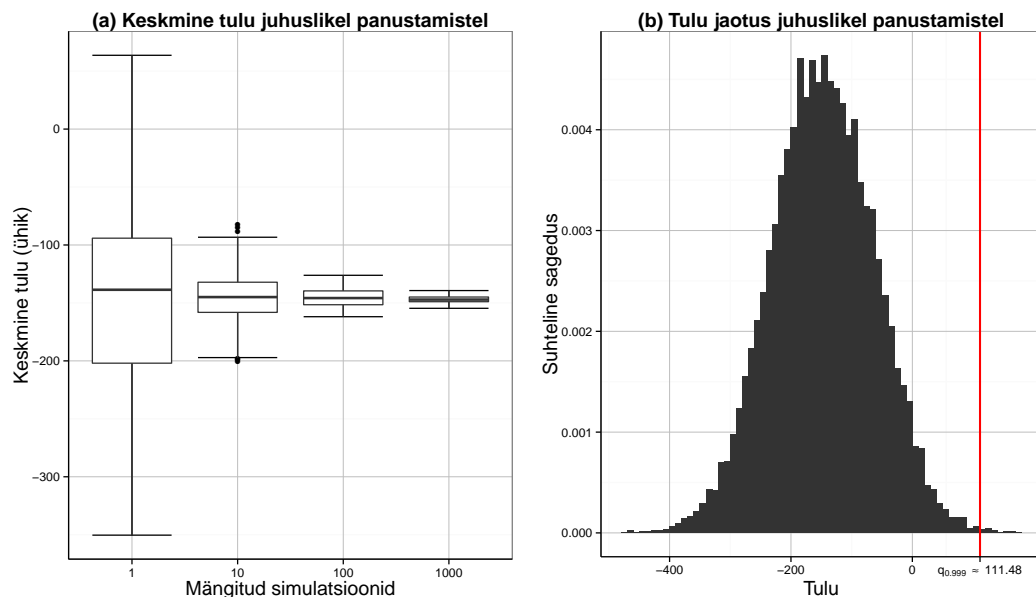
Joonis 5.1: (a) Keskmise lõpptulu koondumine. Juba 1000 simulatsiooni pealt arvatud lõpptulu keskmine varieerub väikestes piirides, mistõttu võime keskmise kahju suuruse üsna julgelt u 145 ühiku peale hinnata. (b) Lõpptulu jaotuse histogramm 10000 simulatsiooni pealt. Histogramm meenutab väga normaaljaotust. Vertikaaljoonega on tähistatud 99,9%-kvantiil q_{0,999} , mille väärtus on 111,48.
