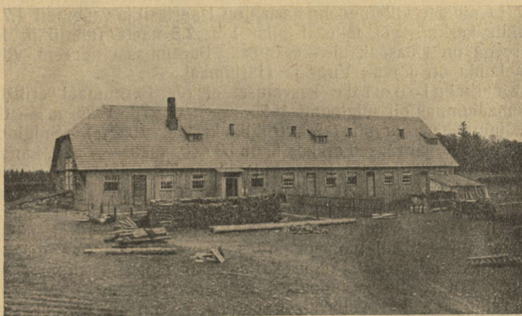
44. joonis. M. Siimu Luba asundustalusavist puhas-karjalaut. Ehitatud 1926. a. ja läks maksma ligi 9000 kr. Et vesi seinu väljast ei leotaks, on seinad laudadega kaetud.
