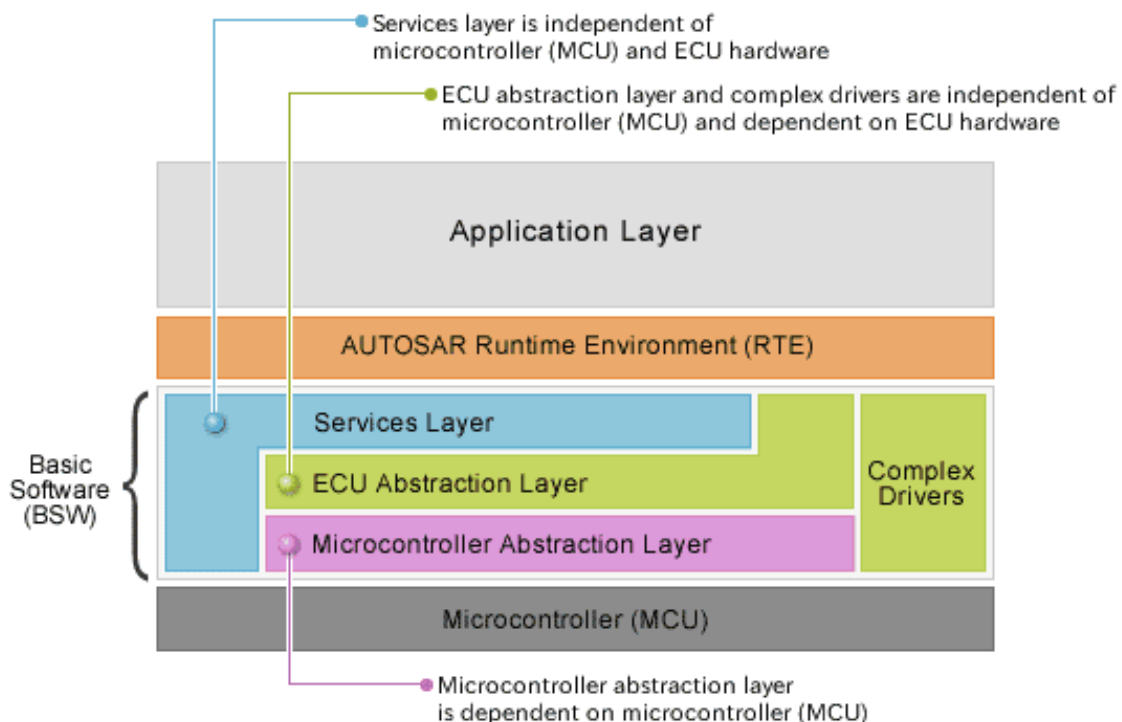
Joonis 2.2: Näide kihelist arhitektuurist: "AUTOSAR Layered Architecture"
