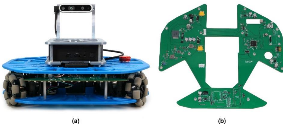
Joonis 3.2: (a) Kokkupandud Robotont 3.0 robot. (b) Robotondi 3.0 emaplaat
