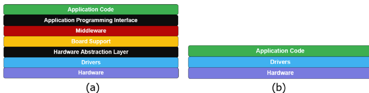
Joonis 2.1: Kihilise arhitektuuri lähenemine. (a) Seitse kihti; (b) Kolm kihti
