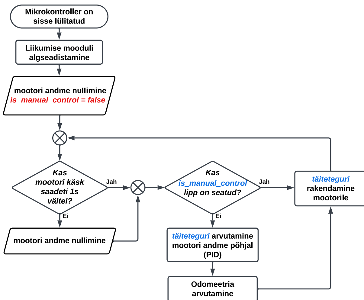
Joonis 5.3: Robotont 3.1 liikumise algoritmi põhitsükkel
