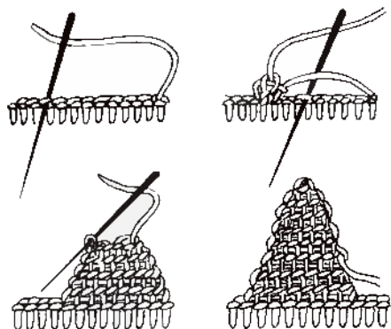
Joonis 42. Hedebotagide tikkimise tehniline joonis ( Allikas: Laanpere & Raidla, 1989 )
