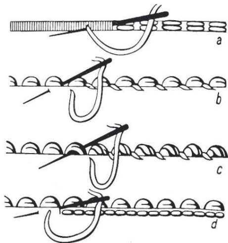
Joonis 23. Liivapistetagide tikkimise tehniline joonis ( Allikas: Linnus 1960)
