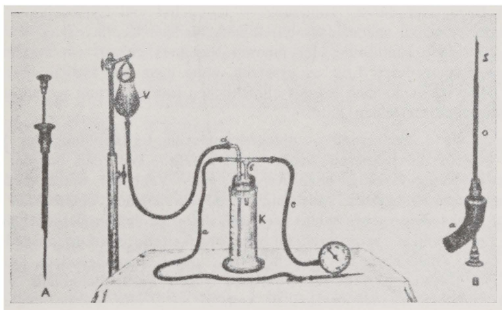
Abb. 60. Apparatur zur Vermeidung von Druckschwankungen bei Ausführung der Ventrikelpunktion.
