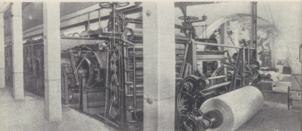
Paberimasin nr. 3. Monteeritud 1922. aastal.
