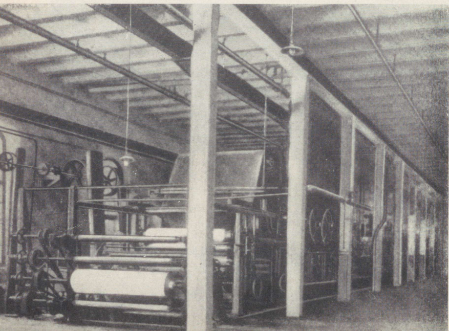
Paberimasin nr. 4. Monteeritud 1914. aastal.
