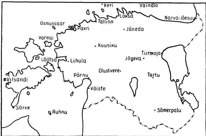
Joonis nr. 11. Lexis'e tegurite arutamiseks kasutatud sademetejaamade asukohad.
