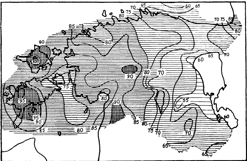
Joonis nr. 5. Keskmine oktoobri samasademejooned (1923—35).
