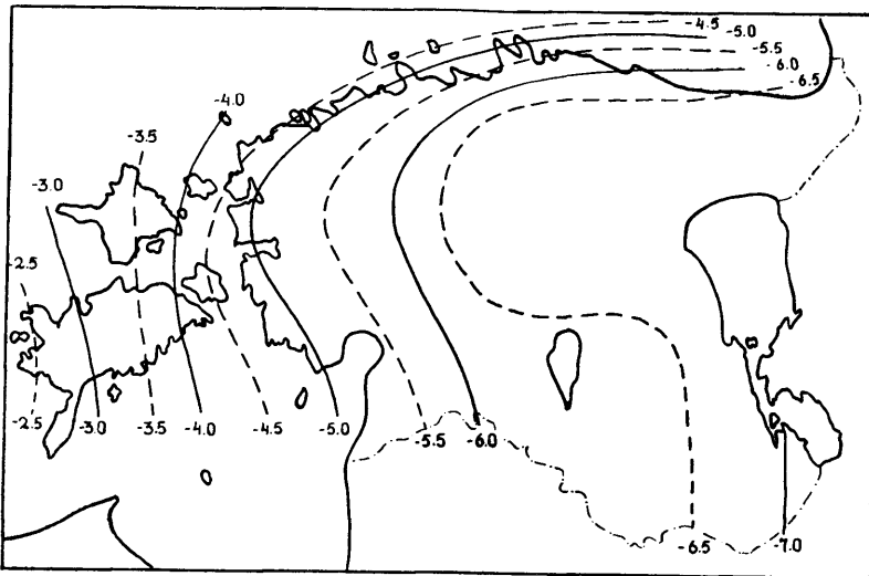
Joonis nr. 1. Jaanuari isotermid (1866—1935).
