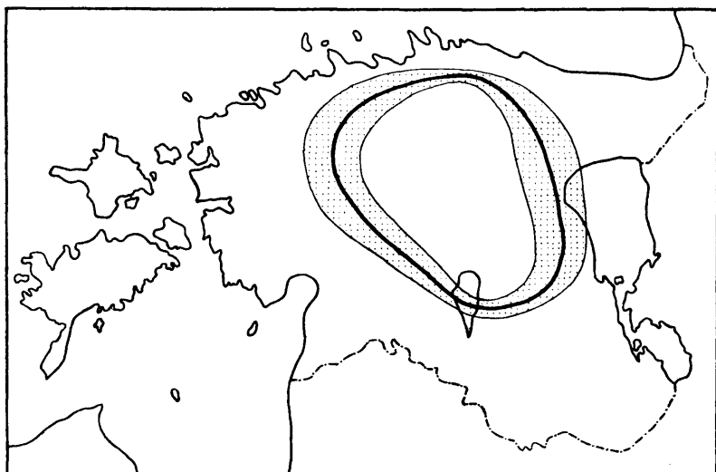
Joonis nr. 9. Sügisesse jahenemise lähte-maaala piirjoon ühes hajumisribaga septembri, oktoobri ja novembri õhutemperatuuri vaatluste järgi.
