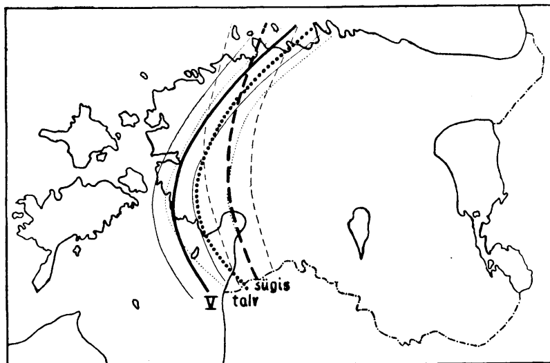
Joonis nr. 3. 0-isanomaalide asendid maikuu, sügiskuudel ja talvekuudel.
