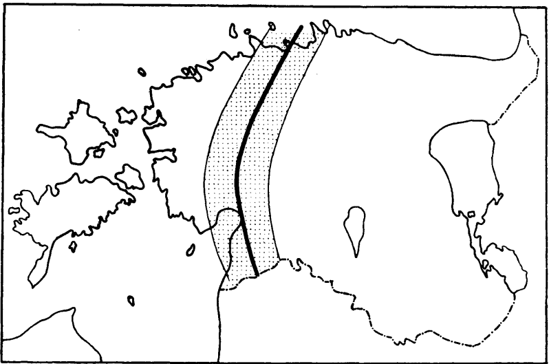
Joonis nr. 7. Kliima-valdkondi lahutav piirikõver ühes hajumisribaga.
