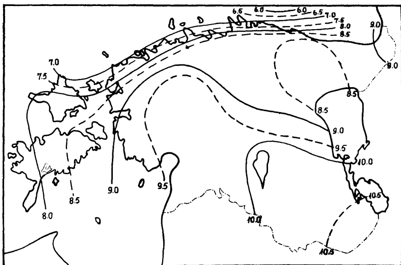
Joonis nr. 2. Mai isotermid (1866—1935).
