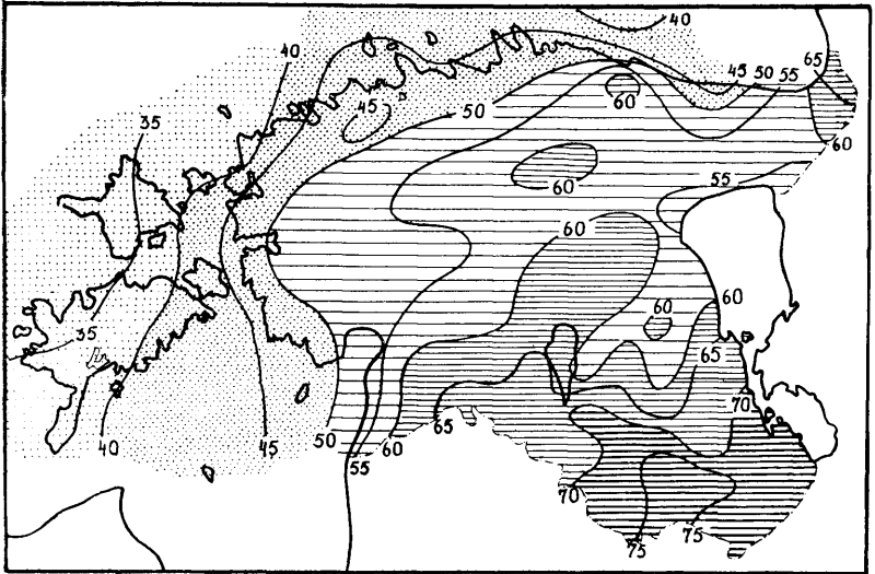
Joonis nr. 4. Keskmine juuni samasademejooned (1923—35).
