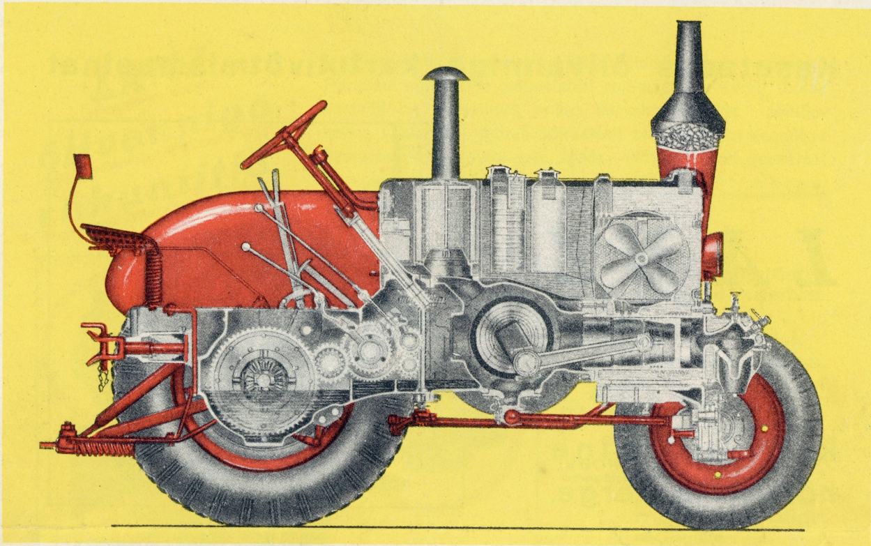
Pikkiläbilõige LANS Bulldog traktorist. 6 käiguga ja elektriseadeldisega.
