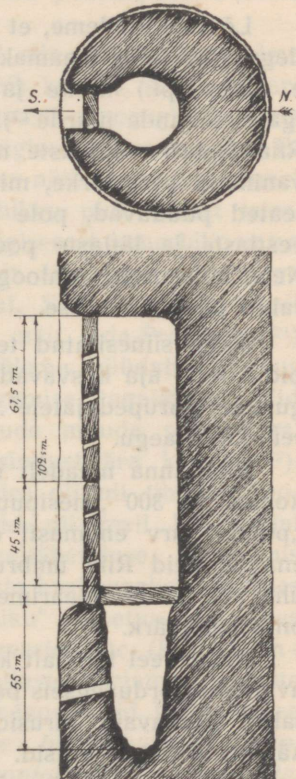
Joon 2. Eelmise „tarupedaja“ pesaruumi läbilõiked.
