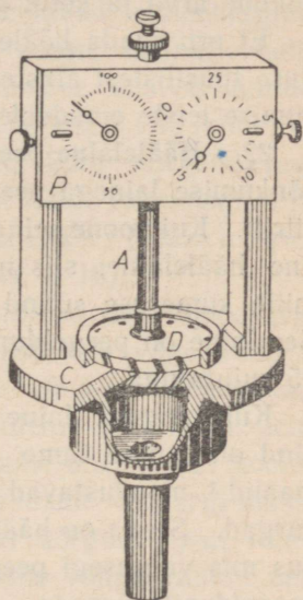
Joon. 29. Cagniard de la Tour'i sireen.
