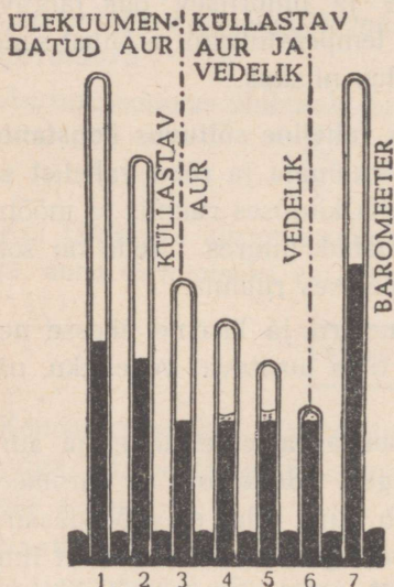
Joon. 99. Auru rõhu muutumine sõltuvalt ruumala muutumisest ja mitteküllastava auru üleminek teataval temperatuuril küllastavaks auruks.
