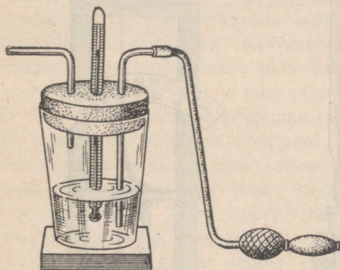
Joon. 106. Lihtsaim hügromeeter.
