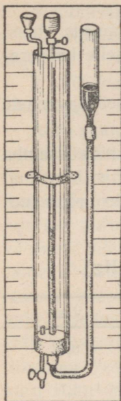
Joon. 101. Katseriist auru rõhkude mõõtmiseks mitmesuguste temperatuuride puhul.
