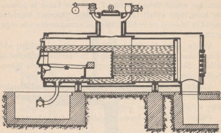
Joon. 115. Suitsutoru-aurukatel.
