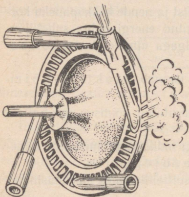
Joon. 124 Auru käik auruturbiinis.
