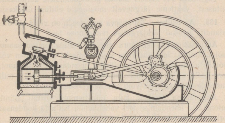
Joon. 118. Kahepoolse tegevusega aurumasina skeem.
