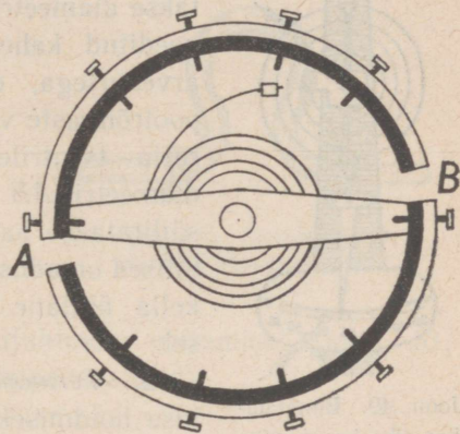
Joon. 48. Kella kompensatsioon-balanssratas.
