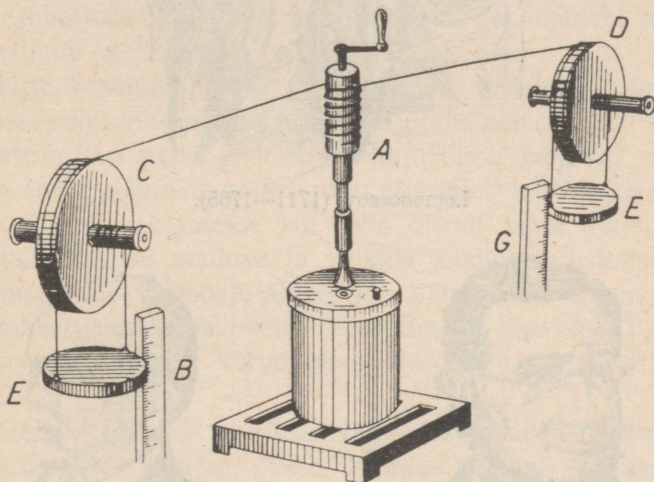
Joon. 42. Joule'i katseseade soojuse mehaanilise ekvivalendi määramiseks.
