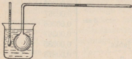
Joon. 62. Dilatomeeter.
