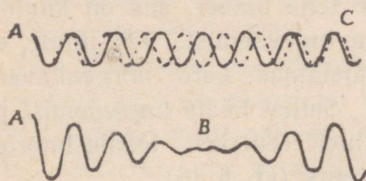
Joon. 30. Tuiklemiste tekkimine.
