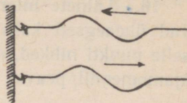
Joon. 13. Peegeldumine poollaine kaotusega.
