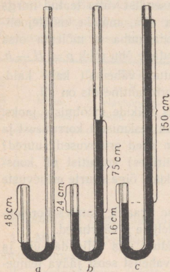
Joon. 59. Gaasi ruumala väheneb rõhu suurenemisega.
