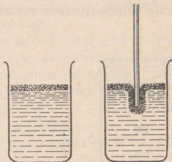
Joon. 75. Rasvatud klaaspulk vette laskmisel painutab pinnakelmet.
