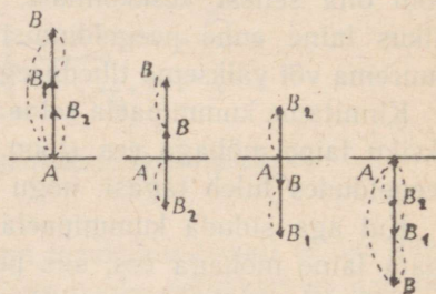
Joon. 16. Nihete algebralise liitmise neli juhtu.
