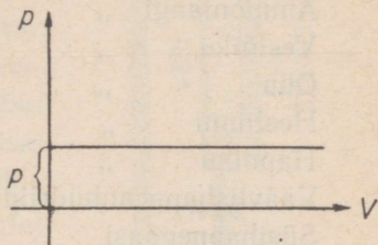
Joon. 63. Isobaar.
