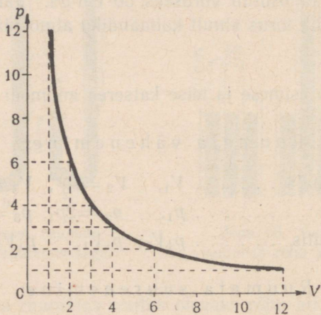
Joon. 61. Gaasi rõhu sõltuvuse graafik ruumalast.
