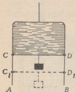
Joon. 71. Pinget kelme piiril võib tasakaalustada vihi kaaluga.
