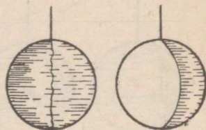
Joon. 73. Kelme pin- ge tõmbab niiti pingule kaart mööda.
