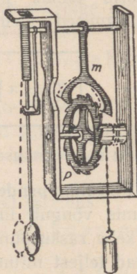
Joon. 5-a. Kella käigu reguleerimine pendli abil.
