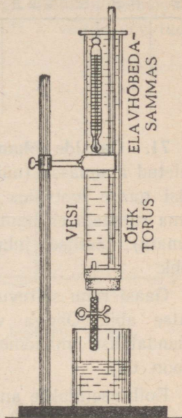
Joon. 64. Katseriist laboratoorse töö nr. 8 juurde.
