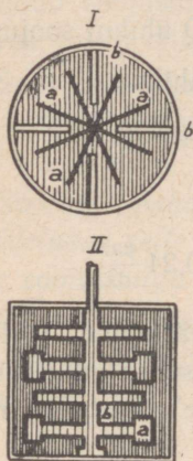
Joon. 41. I — Joule'i kalorimeetri horisontaalne läbilõige, II — vertikaalne läbilõige.
