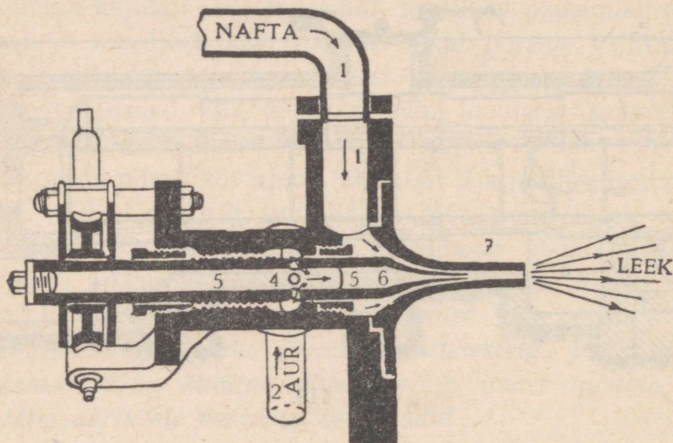
Joon. 114. Pihusti.
