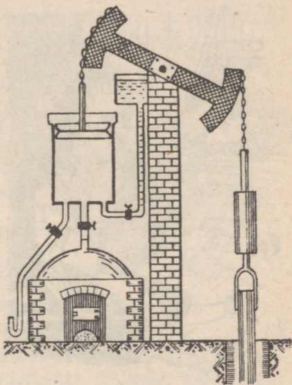
Joon. 117. Newcomeni aurumasin skeem.
