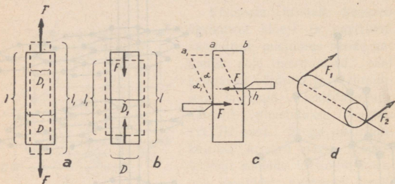
Joon. 91. Deformatsiooni põhiliikide skeem.
