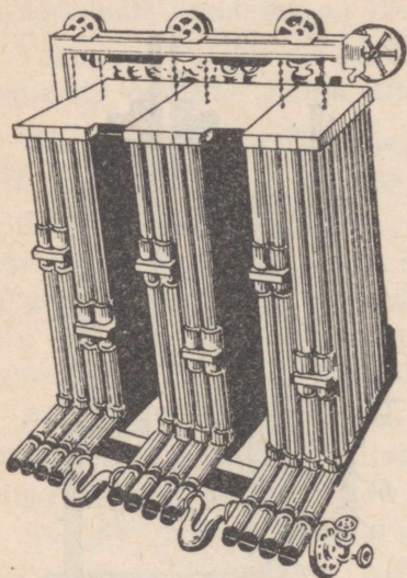
Joon. 120. Ekonomaiseri.
