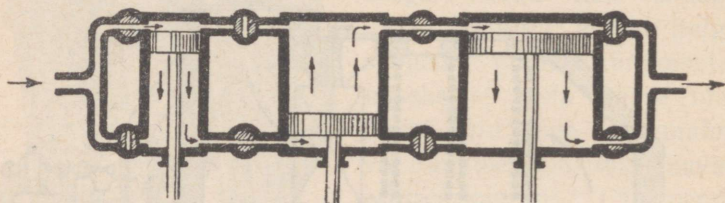
Joon. 122. Kolmekordse paisutamisega aurumasina skeem.
