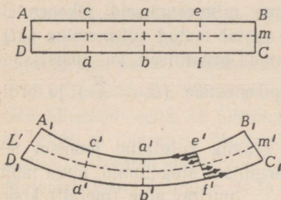
Joon. 94. Deformatsioon painde puhul: punktiirjoon on neutraalne kiht, noolekesed lõikes e'f' on selles lõikes mõjuvad välisjõud.
