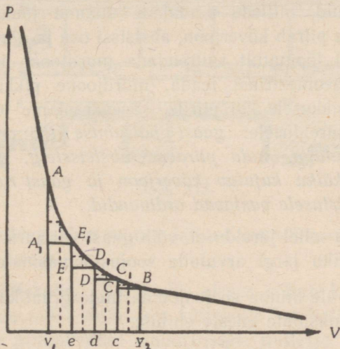
Joon. 112. Gaasi paisumise töö mõõtmine gaasi oleku muutumise graafiku järgi.
