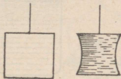
Joon. 72. Kelme pin- ge kisub ristküliku nii- dist küljed sissepoole.
