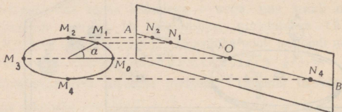
Joon. 3. Liikuva raadiuse pöördenurka ( \alpha ), mille ta moodustab raadiuse algasendiga, nimetatakse võnkefaasiks.
