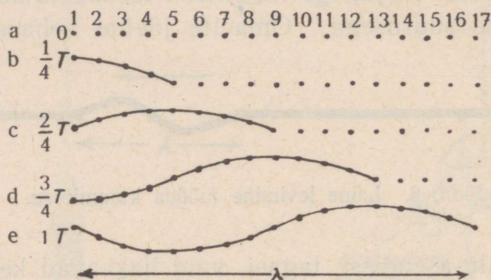
Joon. 9. Ristvõnkumise levimine.
