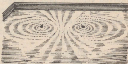
Joon. 19. Lainete interferents vee pinnal.
