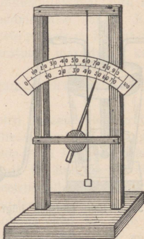
Joon. 109. Juushügromeeter.
