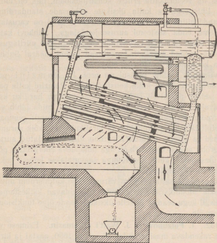
Joon. 116. Veetoru-aurukatel.
