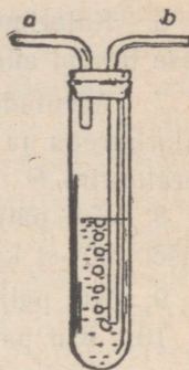
Joon. 104. Aurukuivataja.
