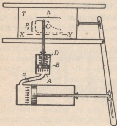
Joon. 123. Watt'i indikaatori ehituse ja töötamise skeem.
