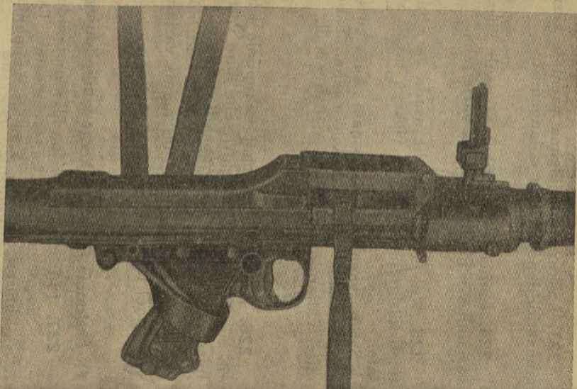
Bild 13. Verkürzter Trageriemen zum Schießen während der Bewegung. Pilt 13. Lühendatud kanderihm laskmiseks liikumisel.
