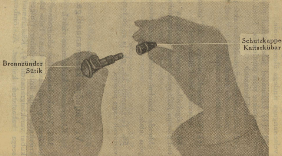
Bild 6. Abschrauben der Schutzkappe vom Brennzünder der Eihandgranate. Pilt 6. Kaitsekübara ärakruvimine muna-käsigranaadi sütikult.
