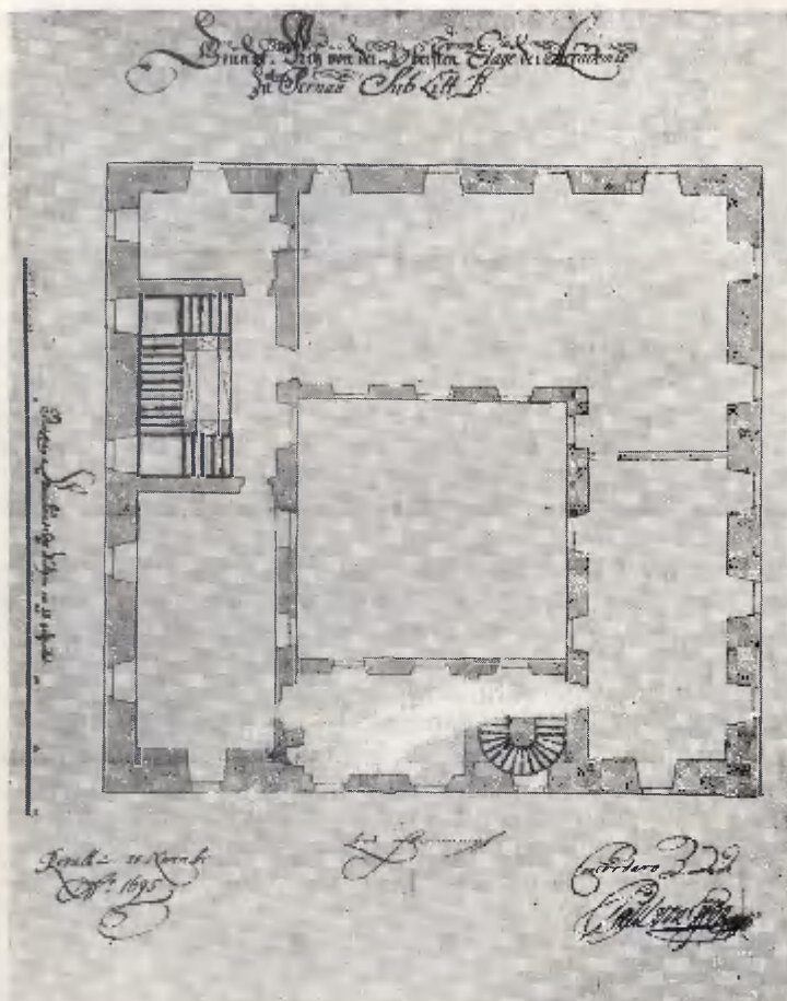
Bild 13. Akademien i Pärnu. Plan av övre våningen. (Kammararkivet, Stockholm.)
