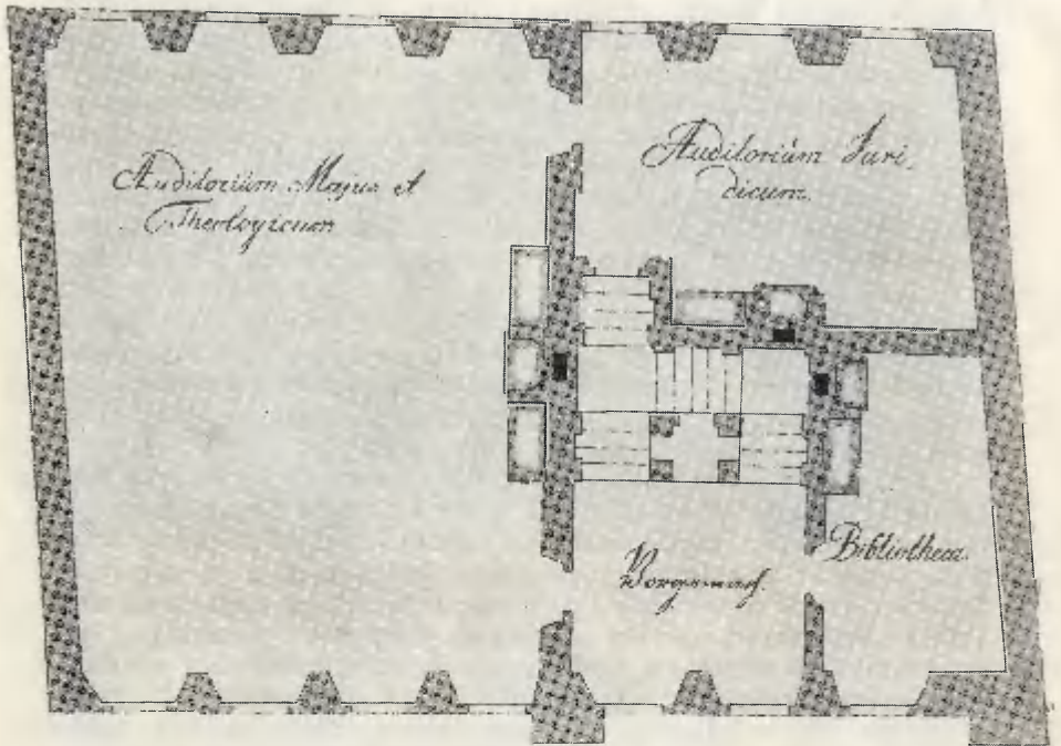
Bild 8. 1690 års universitetshus i Tartu. Plan av övre våningen. Ritning av P. von Essen. (Dommuseum, Riga.)
