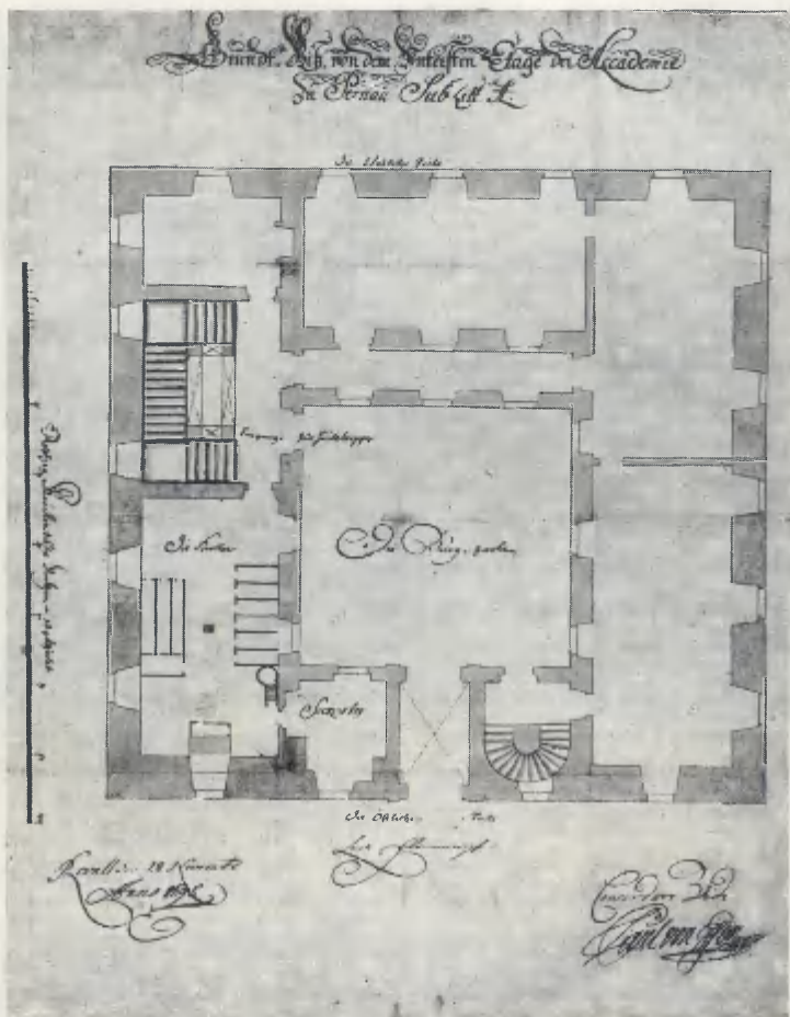
Bild 12. Akademien i Pärnu. Plan av första våningen. (Kammararkivet, Stockholm.)
