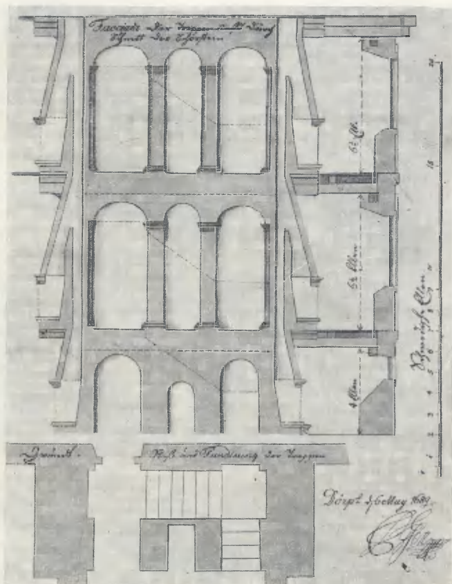
Bild 9. 1690 års universitetshus i Tartu. Sektion och plan av trapphuset. Ritning av P. von Essen. (Dommuseum, Riga.) Ülikooli hoone 1690. a.: trepihoone läbilõige.
