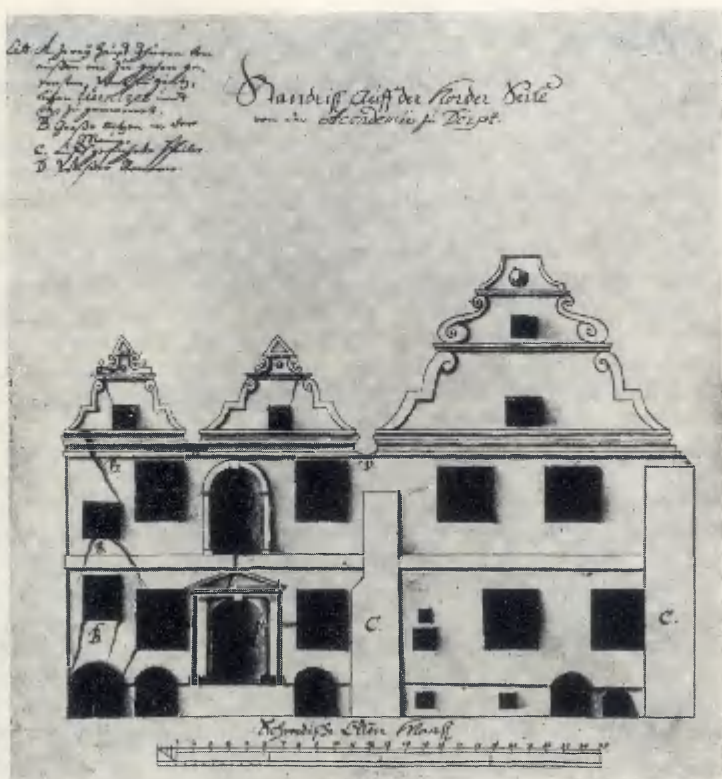
Bild 3. 1640 års universitetshus i Tartu. Fasad. Ritning av P. von Essen 1688. (Riksarkivet, Stockholm.)
