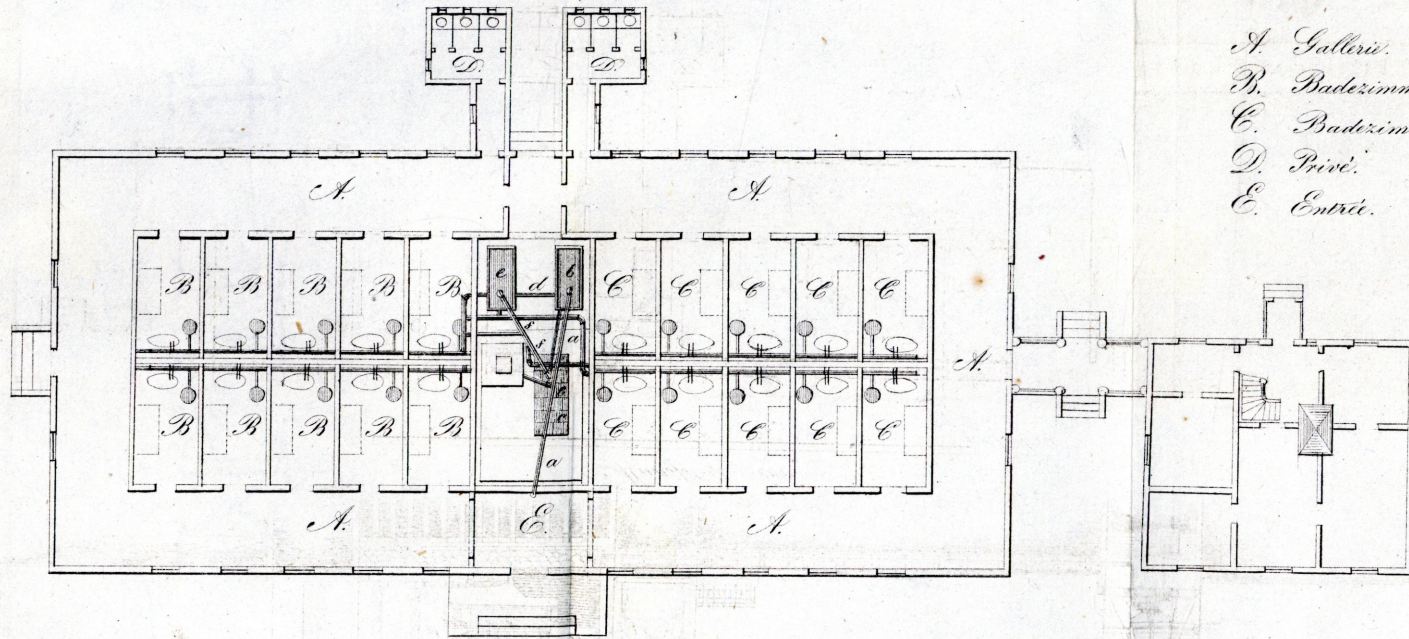
Grundriß
