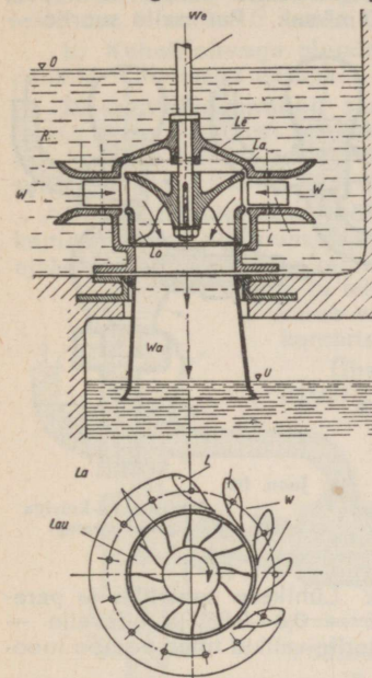
Joon. 15. Fraansisturbiin.
