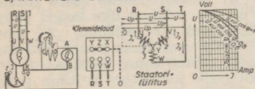
b) KOLMNURK-STAATOR
