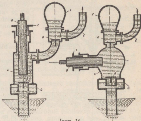
Vertikaal-kolviga plunžerpump.
