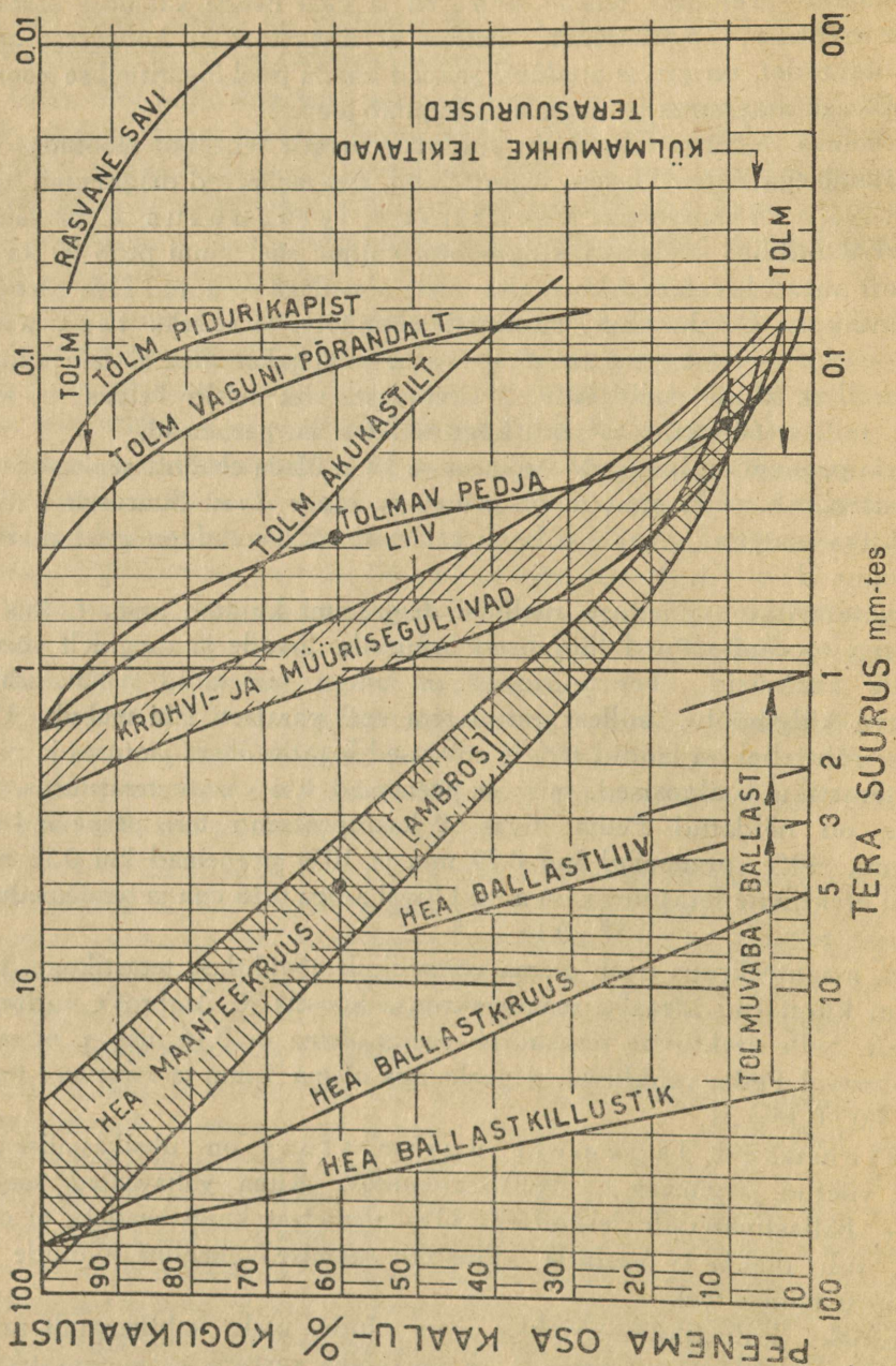
Joon. 1. Tüüpiliste liivade, kruusade ja killustiku terasuuruse diagramm.
