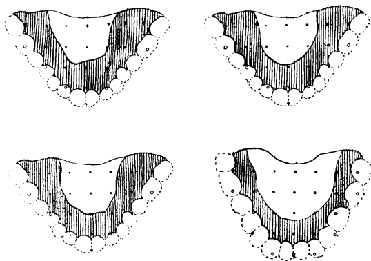
Pilt 7. Palatogramme sõnast udü .
