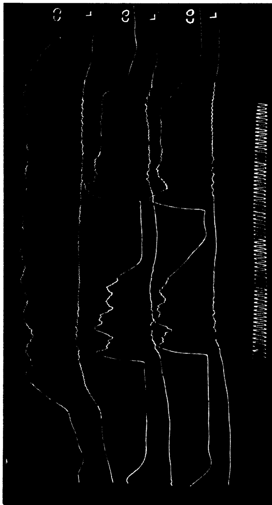
Pilt. 5. Ülemised suu-(CO) ja kõrisõlme-(L) kurvid kujutavad külmaväljendist \bar{\psi} . Alumised kurvid on kahekordsest hobuse peatamisest: \psi\psi . Hääldeaja: teatrikooliõpilane tartlane.
