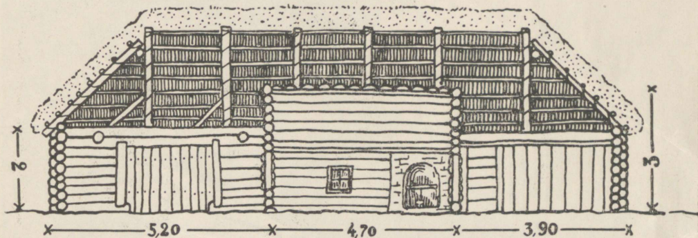
Talumaja piki-läbilõige. Ambla. Keskelt teistest ruumidest kõrgem rehetuba.
