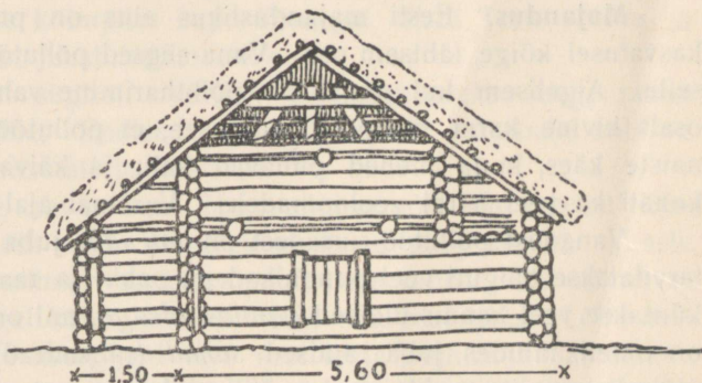
Talumaja rist-läbilõige.
