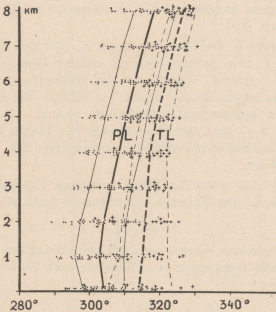
Fig. 4. Vertikale Verteilung der äquivalent-potentiellen Temperaturen in PL und TL im Sommer.
