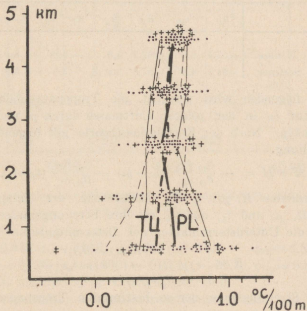
Fig. 10. Vertikale Verteilung des Temperaturgradienten \gamma in PL und TL im Sommer.
