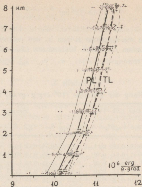
Fig. 5. Vertikale Verteilung der Entropie in PL und TL im Winter.
