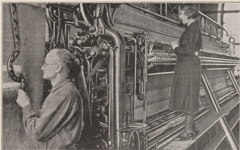
Gipüürpitsi masin töö.
