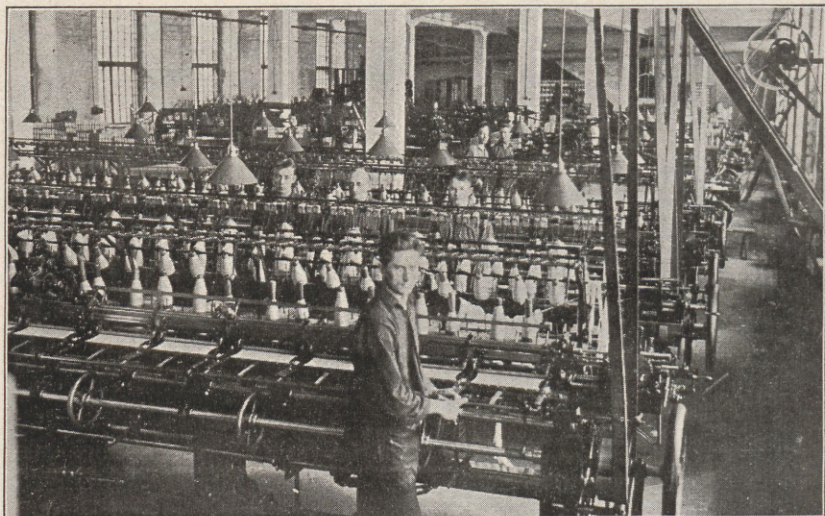
Cotton-suka ja gipüürpitsi masinate saal.
