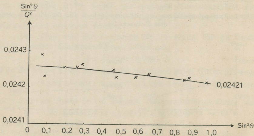
Abb. 8. Extrapolationskurve der Gitterkonstante für die Phase D von dem Präparat Nr. 12.
