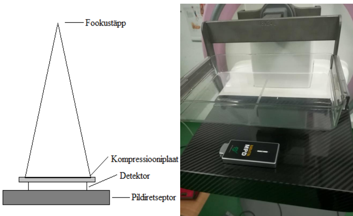
Joonis 6. Kalibreerimise katseskeem.
