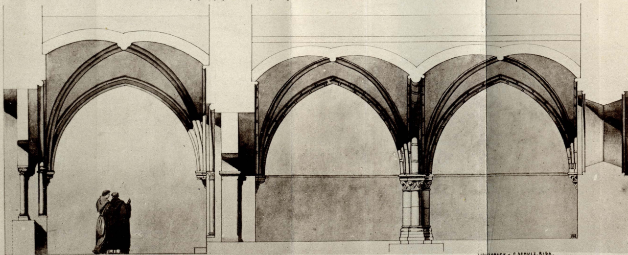
QUERSCHNITT DURCH KREUZGANG UND CAPITELSAAL [G-H].
