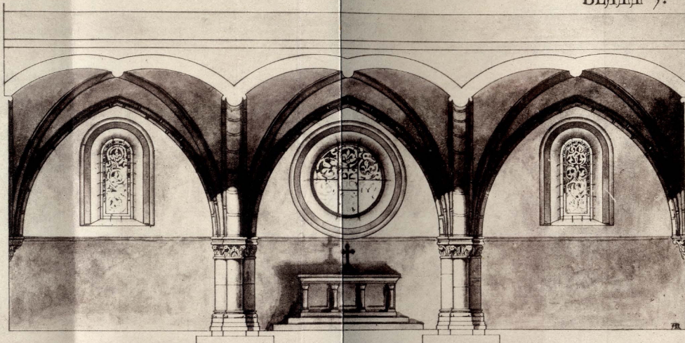
LÄNGSSCHNITT [A-B].
