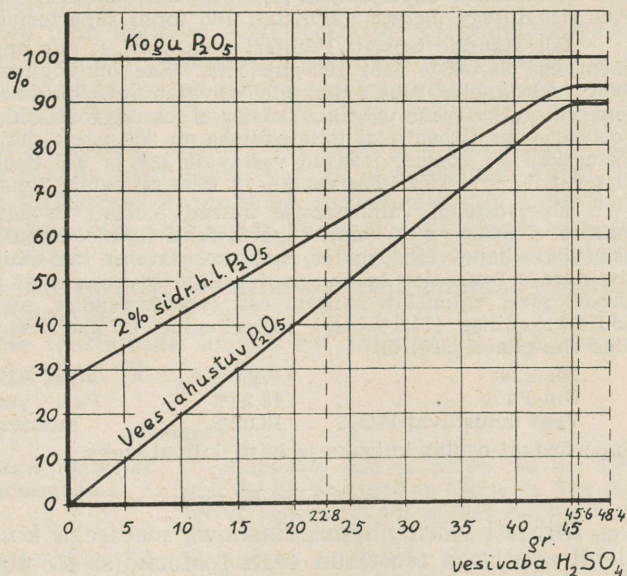
Graafik 3. P_2O_5 lahustuvaks muutumise määra sõltuvus 62%-lise väävelhappe hulgest.
