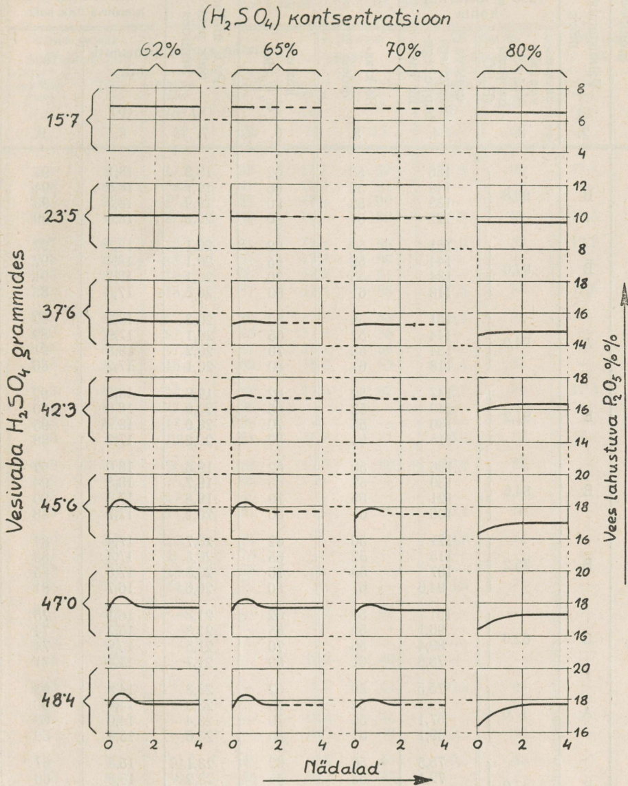
Graafik 1. Vees lahustuva P_2O_5 määrade muutumine eesti fosforiidist valmistatud superfosfaadi proovides aja kestel.
