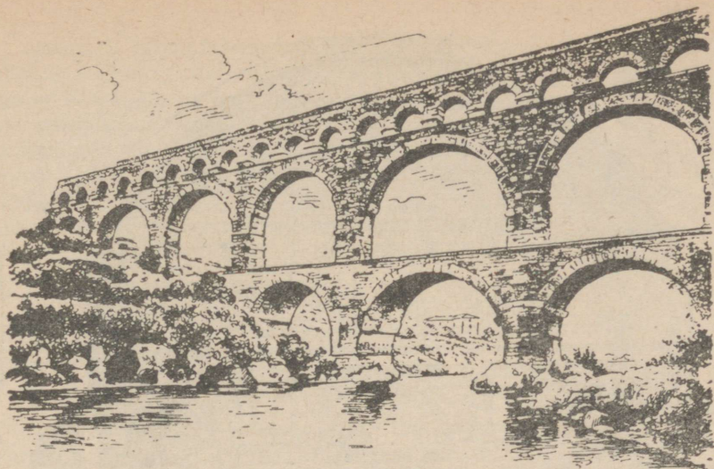
Rooma võlvsild praeguse Prantsusmaa lõunaosas. Silda läbis veevärk. Silla kõrgus jõe veepinnast oli ligi 50 meetrit.
