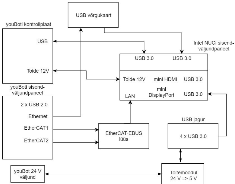
Joonis 8. Intel NUCi ühendused KUKA youBotiga.
