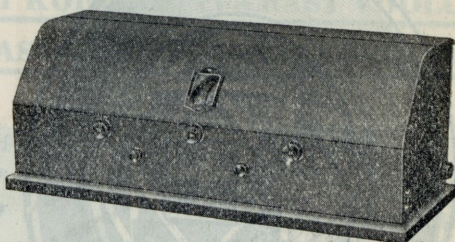
„Tefag 6“ on moodsa lülitusega suurevõimeline vastuvõtja 4-ja astmelise kõrgesagedus-kõvendajaga. Terve aparaat on täielikult kapseldatud. Häälestamine sünnib ainult ühe skaala abil. Suurima kõvenduse saavutamiseks on 1-se lambina tarvitusel kaitsevõre lamp.
