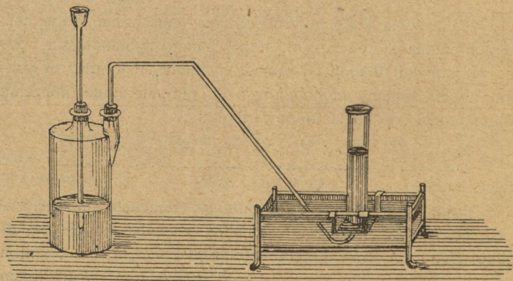
Pilt nr. 24. Wesiniku sünnitamine.
