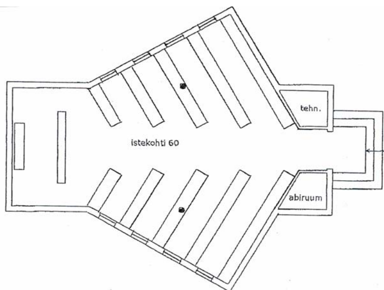
PLAAN 1:100
