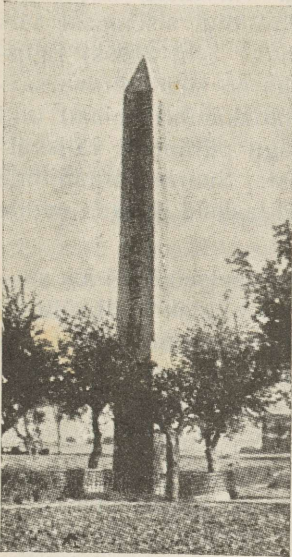
Obelisk.
