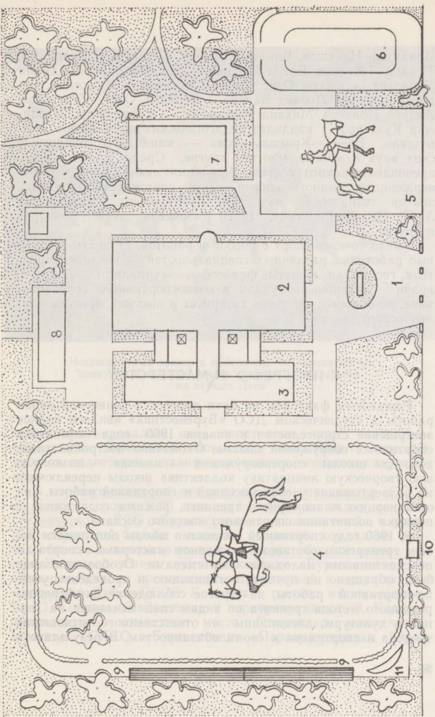
ЭКСПЛИКАЦИЯ: 1. ВХОД, 2. ЗАДАНИЕ МАНЕЖА, 3. КОНЮШНЯ, 4. КОНКУРНОЕ ПОЛЕ, 5. МАНЕЖ ДЛЯ ВЫЕЗДКИ, 6. ШПРИНГЕРТЕН, 7. ОБЩЕЖИТИЕ, 8. ФУРАЖНЫЙ СКЛАД, 9. ТРИБУНЫ, 10. СУДЕЙСКАЯ, 11. ОРКЕСТР.
