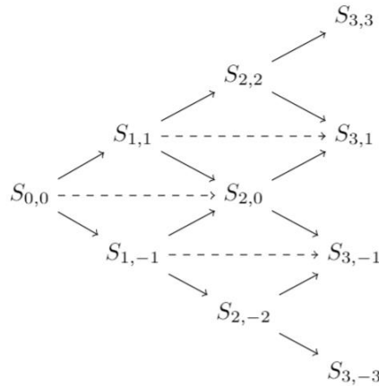
Joonis 4. Alusvara hinnapuu CCS meetodi puhul
