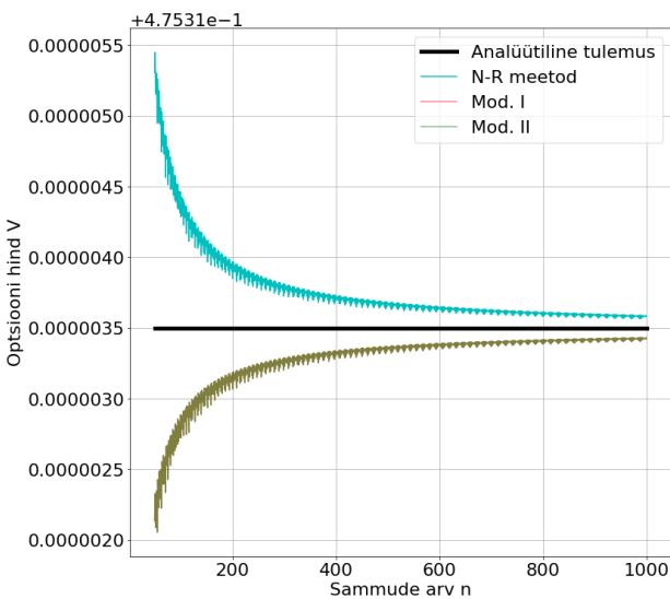
Joonis 9. CCS mod. I, II ja N-R koondumine. \beta = 0,5 ; S_0 = 0,5 .
